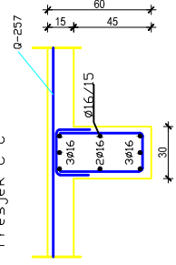
Presjek C-C
