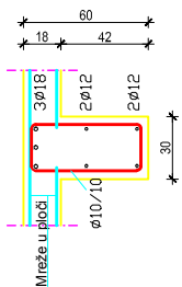
Presjek B-B:
