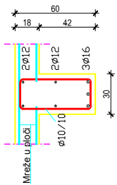
Presjek A-A:
