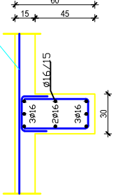
Presjek C-C
