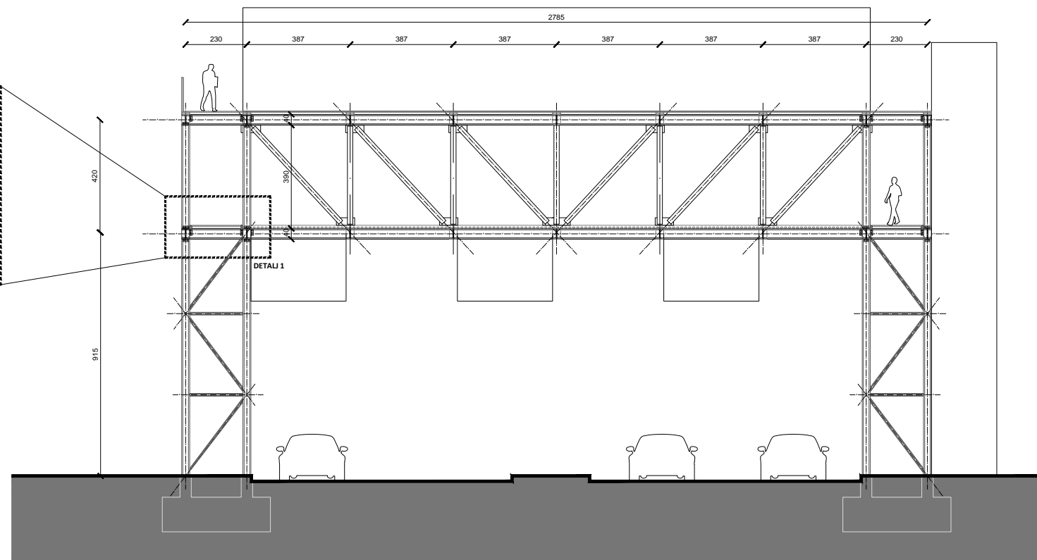
PRESJEK 2-2 M 1:100
