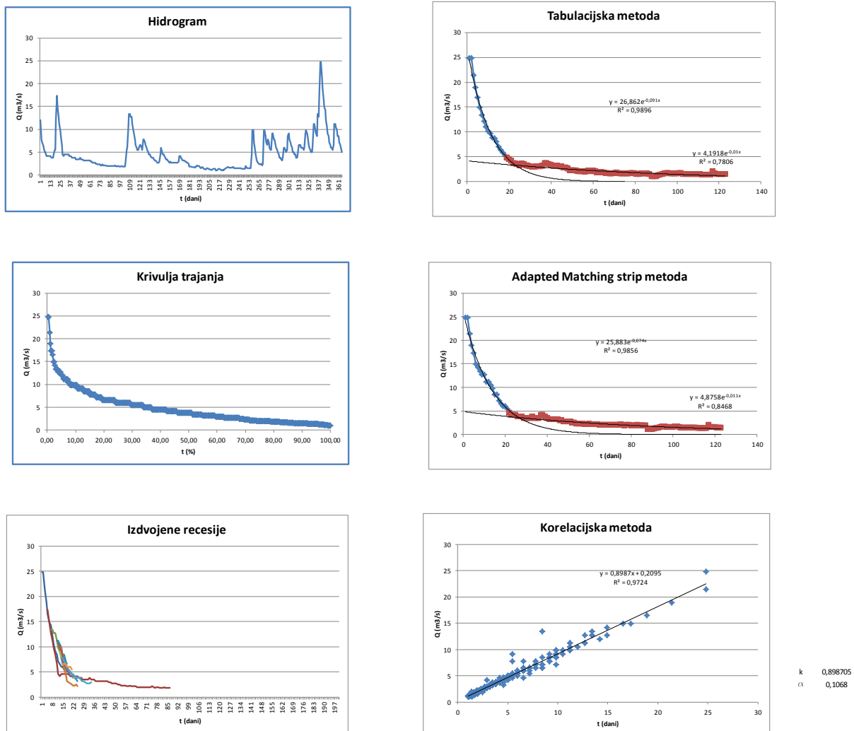
Slika 5.40 Prikaz rezultata analize podataka za 1998. godinu (hidrogram, krivulja trajanja, izdvojene recesije, tabulacijska metoda, „adapted matching strip“ metoda i korelacijska metoda)
