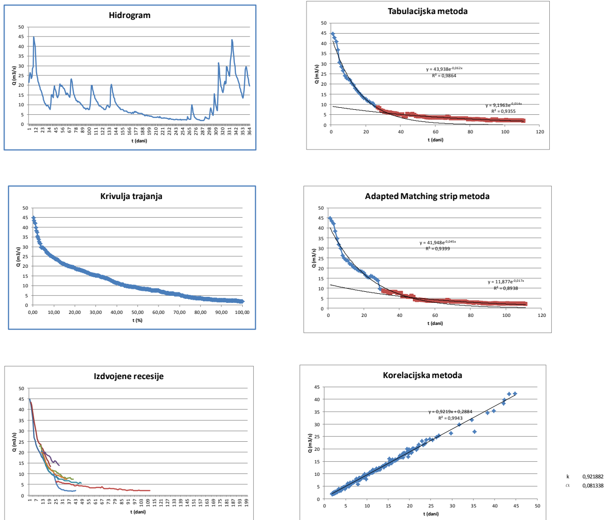
Slika 5.34 Prikaz rezultata analize podataka za 2010. godinu (hidrogram, krivulja trajanja, izdvojene recesije, tabulacijska metoda, „adapted matching strip“ metoda i korelacijska metoda)
