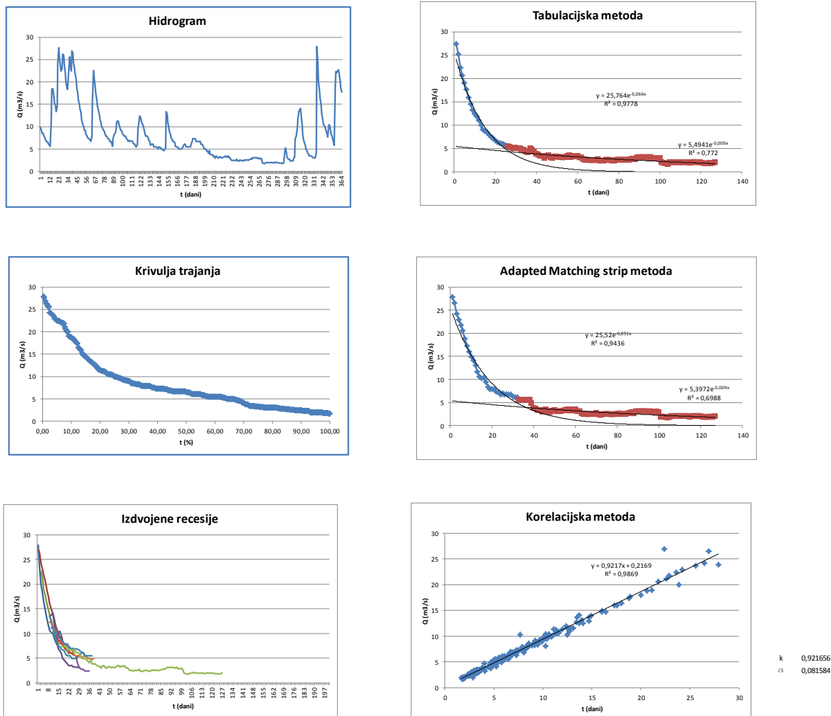
Slika 5.33 Prikaz rezultata analize podataka za 2009. godinu (hidrogram, krivulja trajanja, izdvojene recesije, tabulacijska metoda, „adapted matching strip“ metoda i korelacijska metoda)
