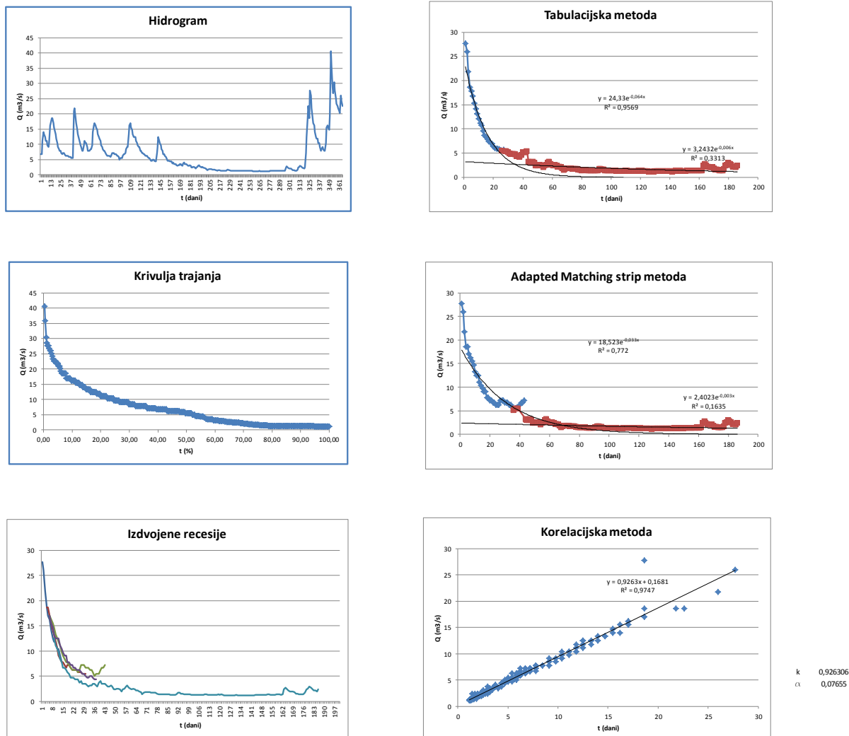
Slika 5.59 Prikaz rezultata analize podataka za 1999. godinu (hidrogram, krivulja trajanja, izdvojene recesije, tabulacijska metoda, „adapted matching strip“ metoda i korelacijska metoda)
