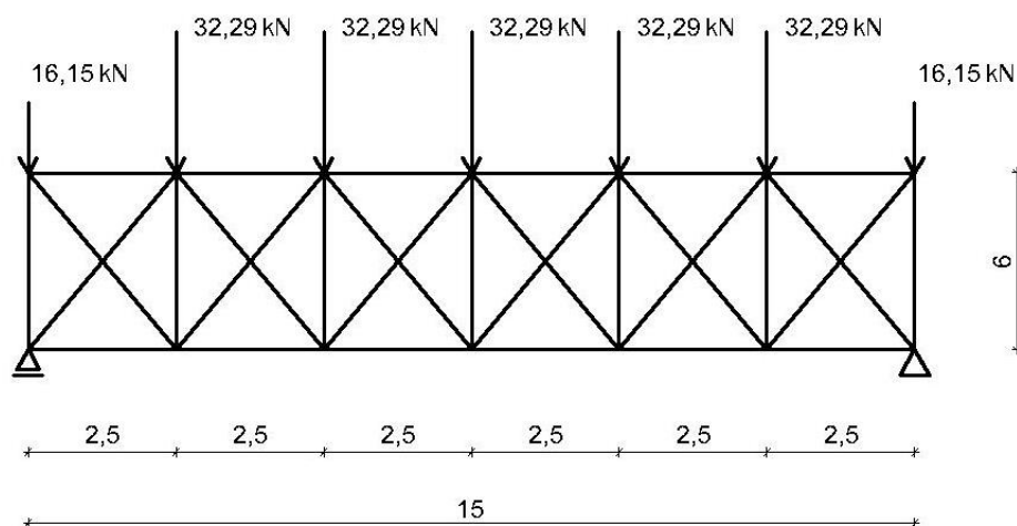
Slika 18 Opterećenje krovnih spregova
