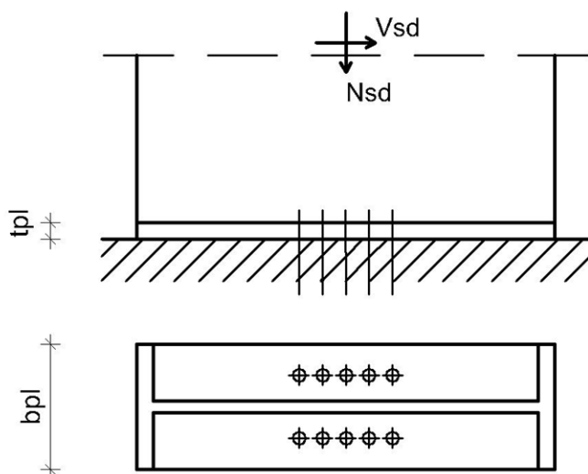
Slika 60 Detalj spoja stup-temelj
