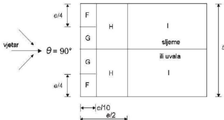
Slika 2.1.2.2.2.3. Prikaz područja vjetra za dvostrešne krovove \Theta=90^\circ
