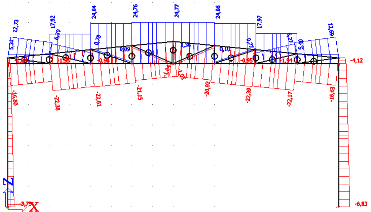
Slika 4.1.3.3. Dijagram uzdužnih sila opterećenja kombinacije 3
