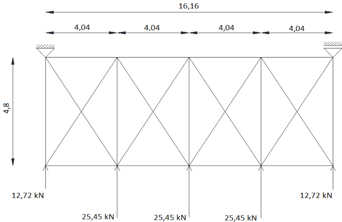
Slika 5.2.1.1. Raspored krovnih spregova i opterećenje
