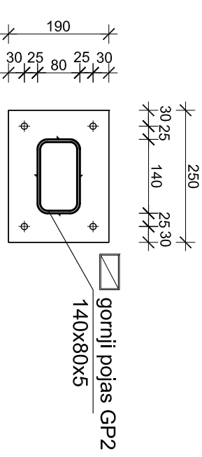
Presjek 5-5
