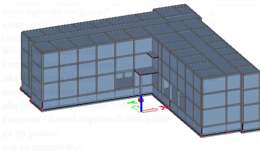
Slika 2.3: Model izrađen u računalnom programu Scia Engineer
