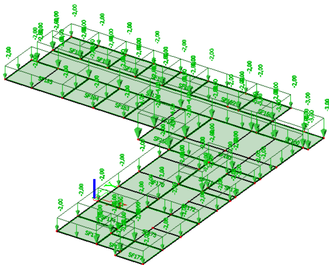
Slika 7.4: Promjenjivo opterećenje Q [ \text{kN/m}^2 ]
