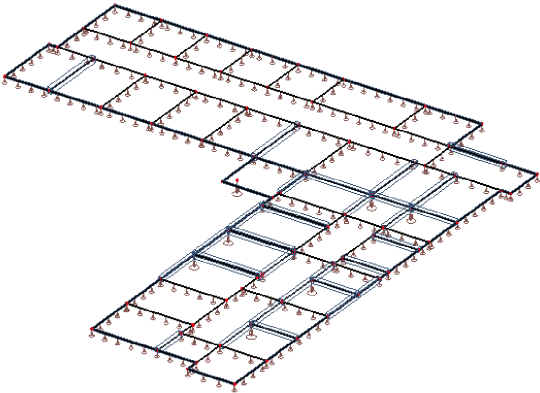
Slika 7.2: Shema ležajeva
