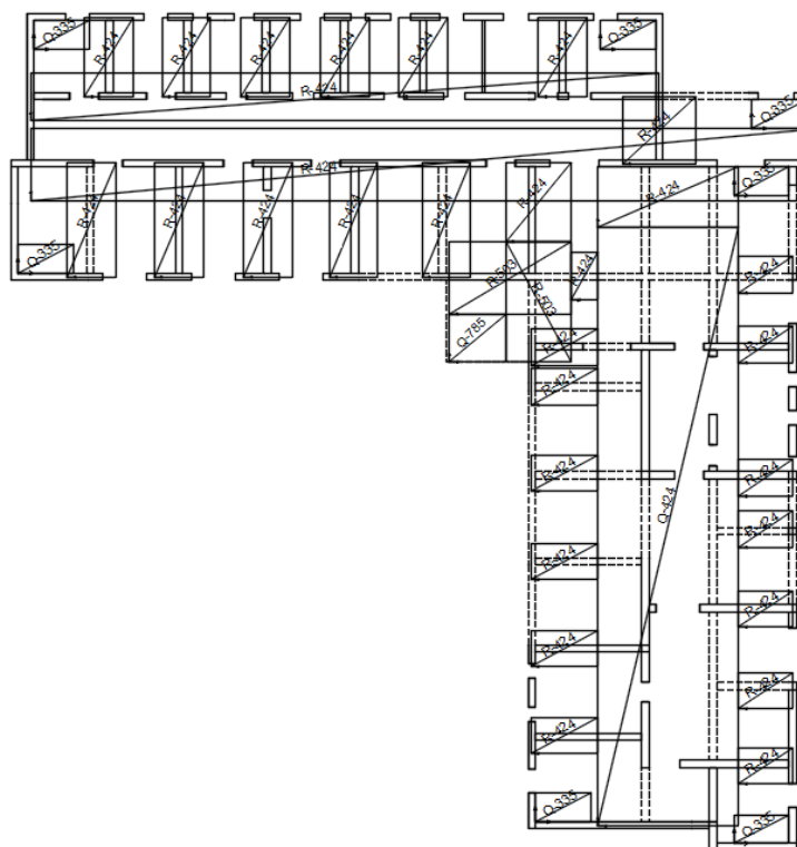
Slika 7.9: Shema armature gornje zone
