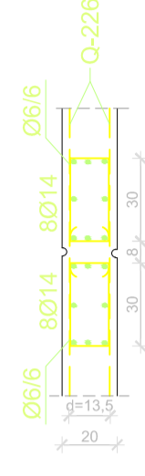
Zid u osi M - detalj F M 1:25
