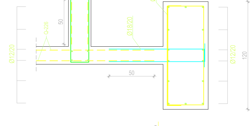
PRESJEK 4 - 4
