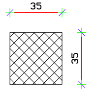
Presjek 1 - 1 M 1:25
