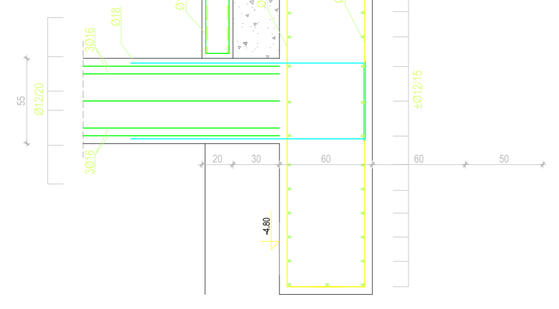
PRESJEK 6 - 6
