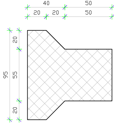
Presjek 1 - 1 M 1:25
