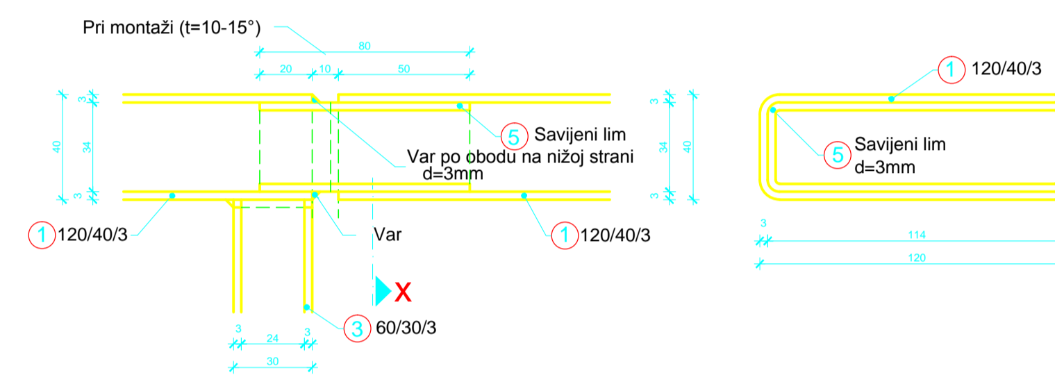
Detalj D1 1:2
