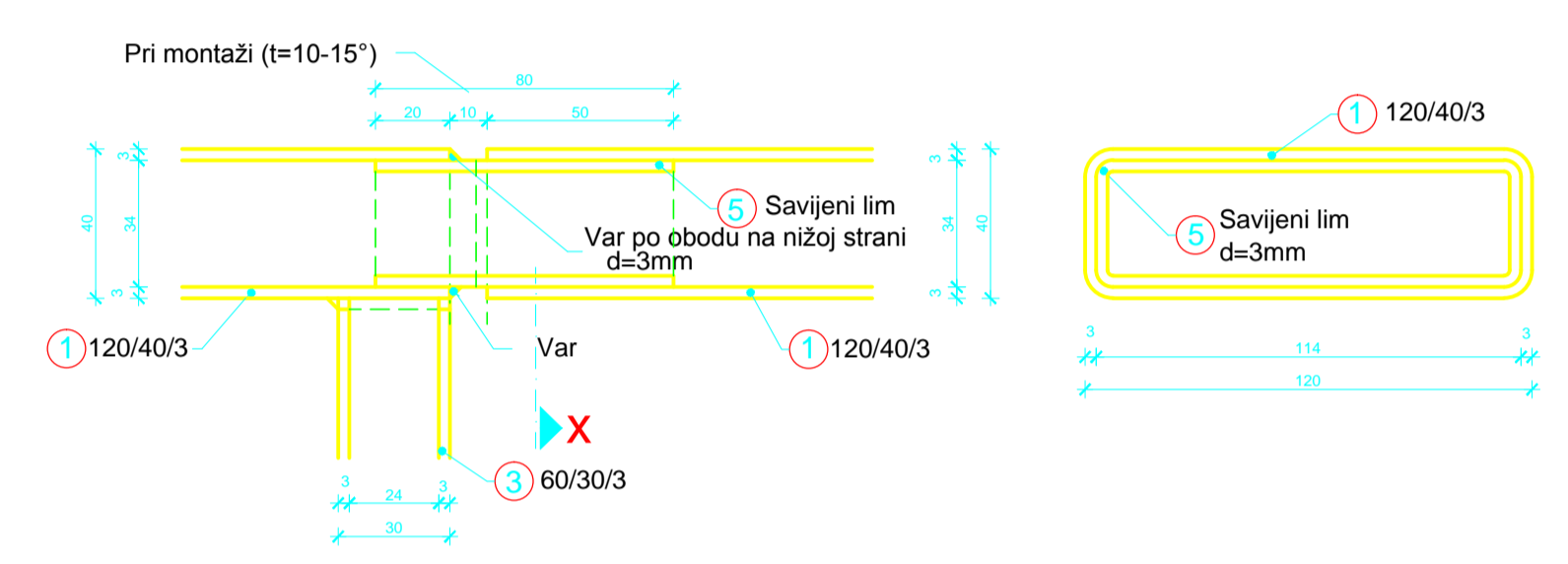
Detalj D1 1:2
