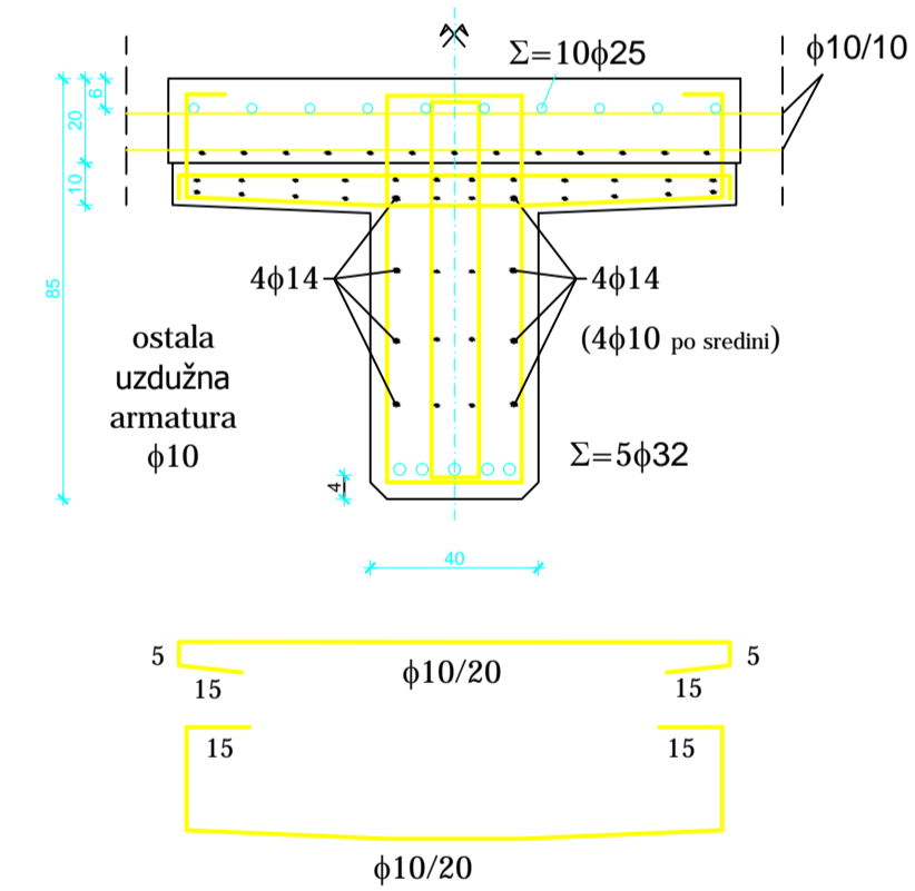
Presjek 2-2
