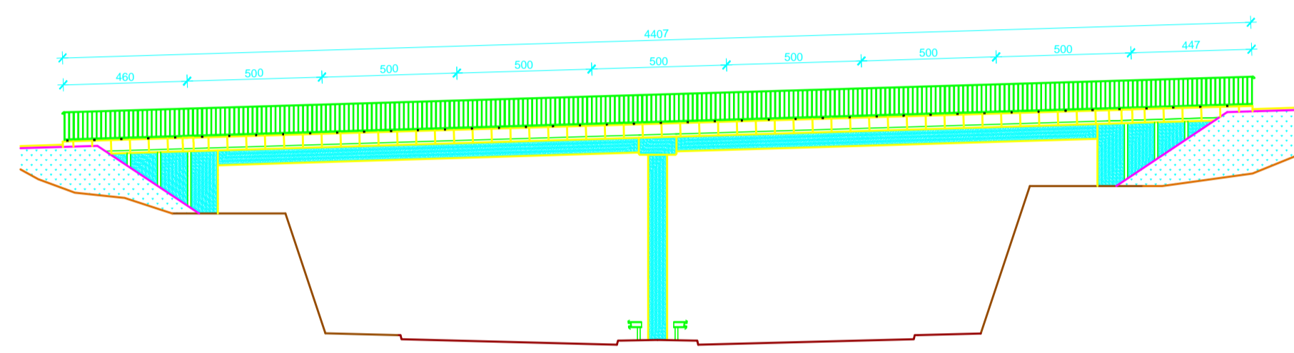
Pogled na most 1:200
