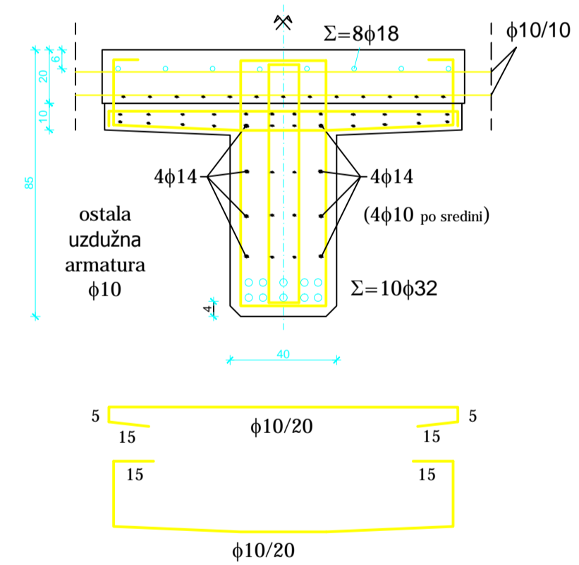
Presjek 1-1
