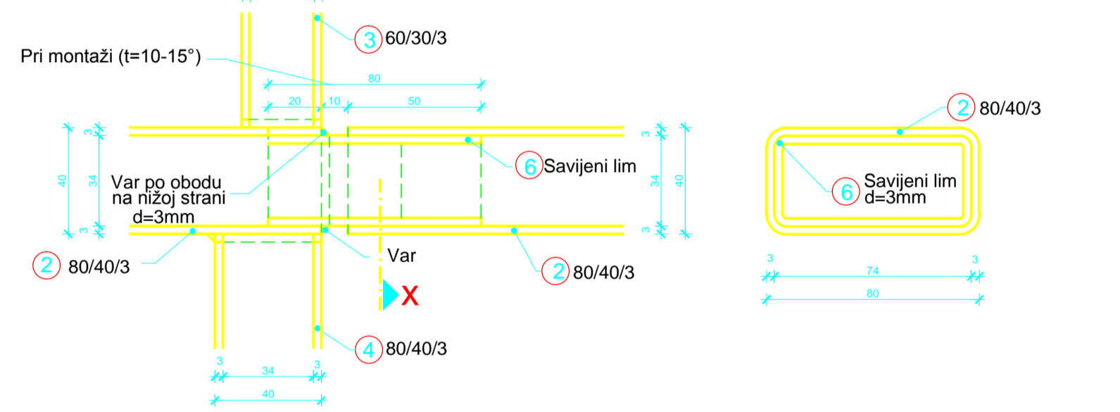
Detalj D2 1:2
