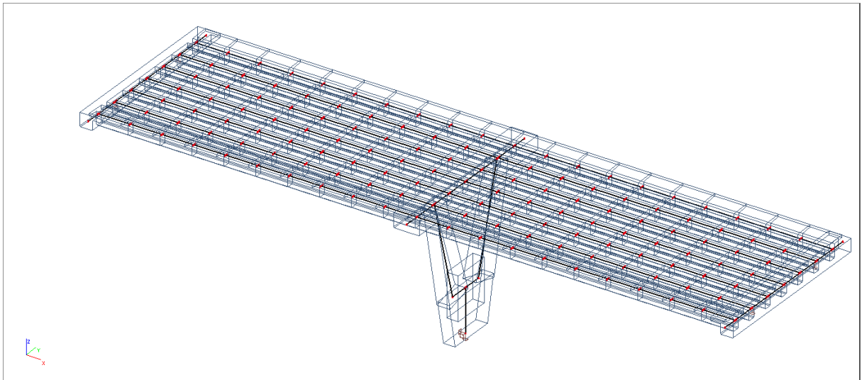
Slika 10 : Stalno opterećenje
