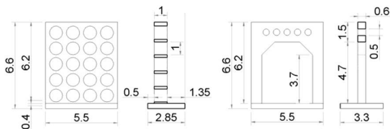
Slika 23. Gradivi elementi lukobrana
