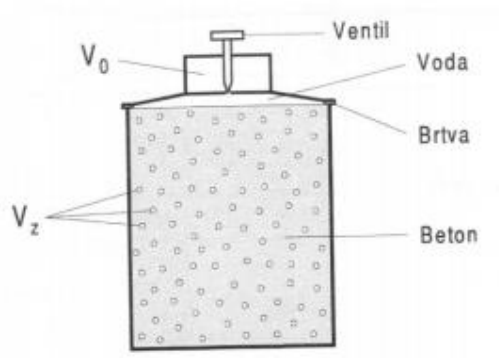
Slika 5.6. Shema manometra [1]
