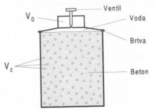
Slika 5.6. Shema manometra [1]
