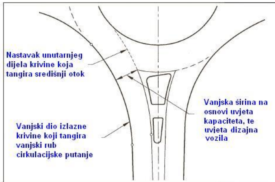
Slika Dizajn izlaska s jednostranog kružnog toka
