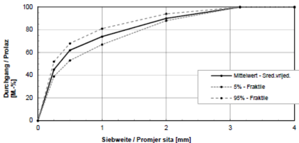
Dijagram 4.2. Granulometrijska krivulja Liapora frakcije 0 – 2 mm [10]
