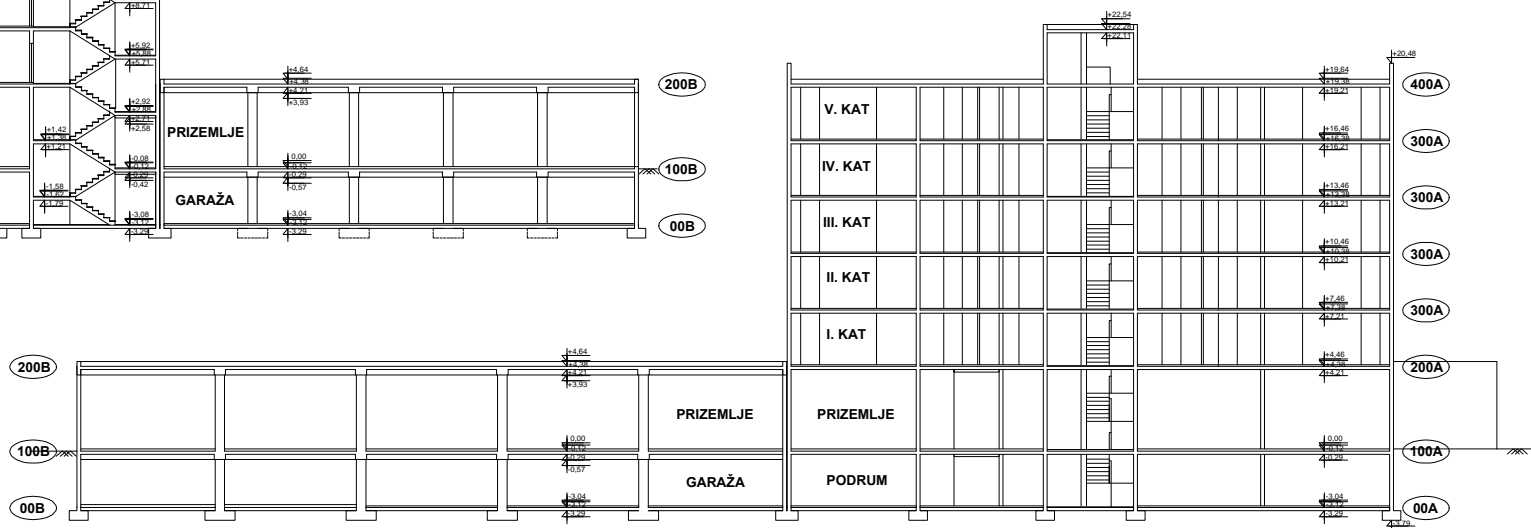
PRESJEK A-A
