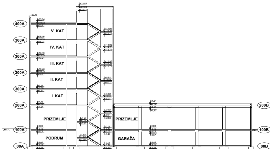
PRESJEK B-B
