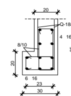
Detalj F
