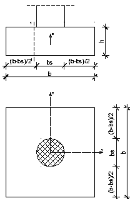
Slika 3.65. Skica geometrije temelja
