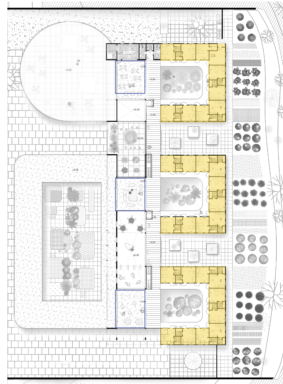
tlocrt kata
