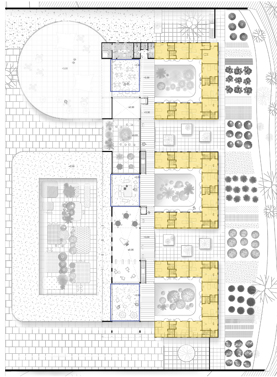
tlocrt kata
