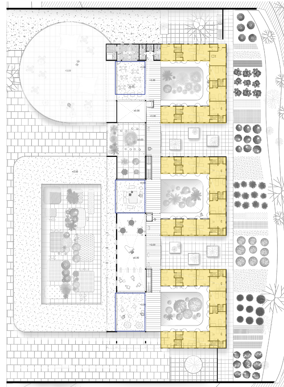
tlocrt kata
