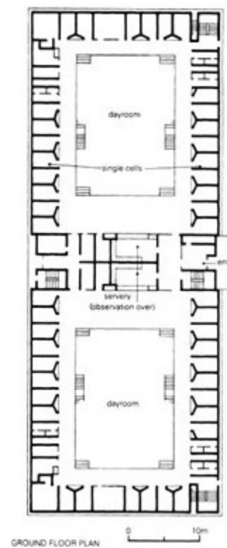
Slika 9: PDBS zatvor (1992), predloženi presjek i tlocrt
