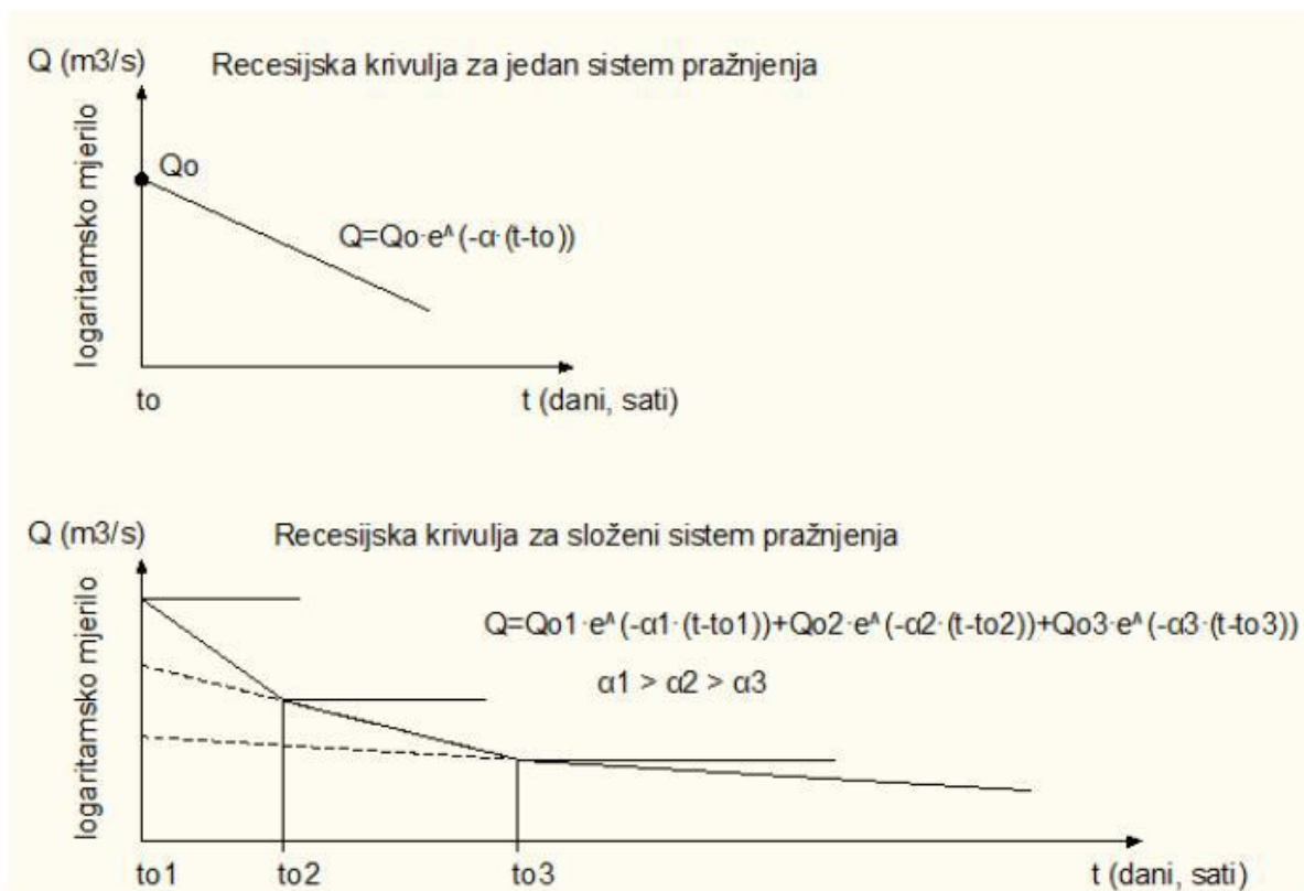
Slika 5.2. Dva tipa reesijskih krivulja (Bonacci)
