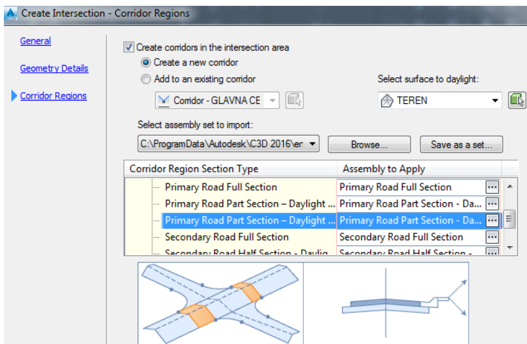
Slika 4.24. Definiranje regija koridora – poprečni presjek desnog traka glavne ceste [9]
