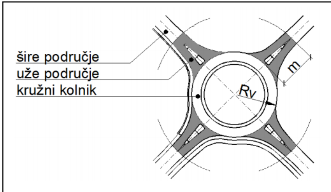
Slika 5.3. Područja kružnog raskrižja [5]
