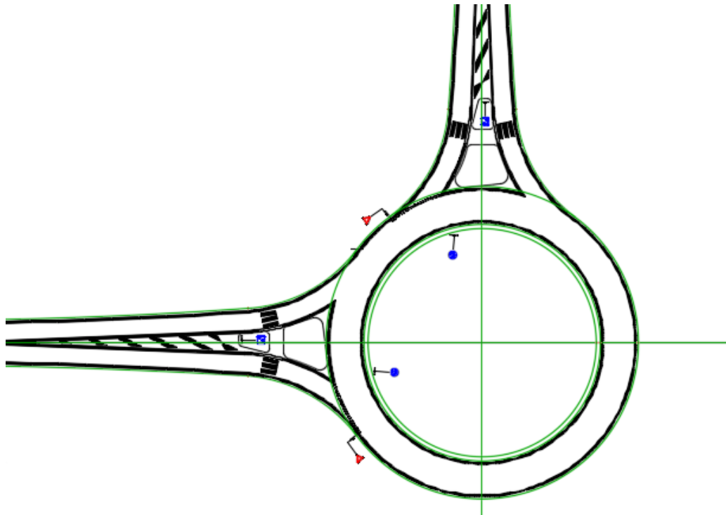
Slika 5.13. Tlocrtni prikaz jednostručnog kružnog raskrižja [9]
