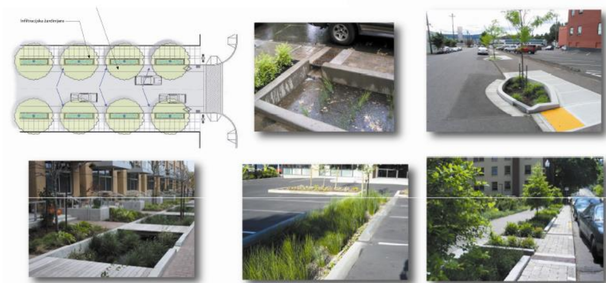
Slika 15.2.3. Mogućnosti odvodnje ulica i parkinga
