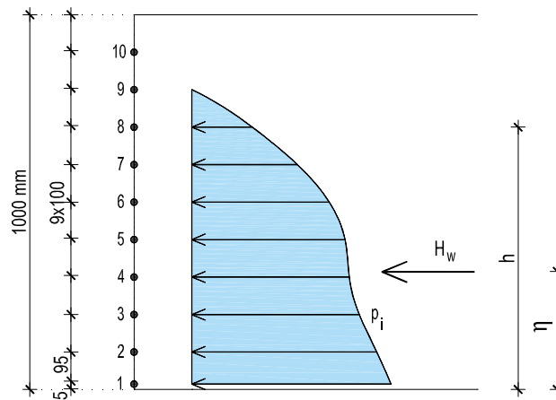
Slika 5.5. Rezultantna sila na čeonu stijenku ( H_w ) i njeno težište ( \eta )
