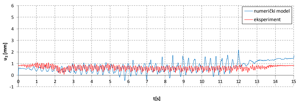
(b) a_0=0.2g
