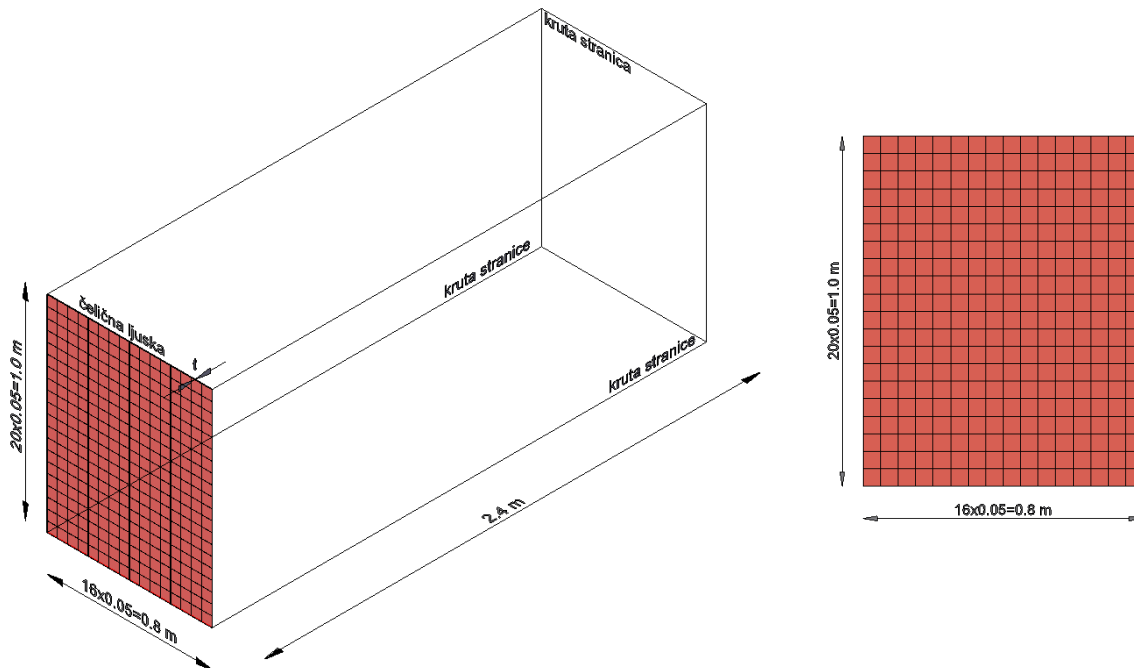
Slika 6.2. Prostorna diskretizacija čelične ljuske
