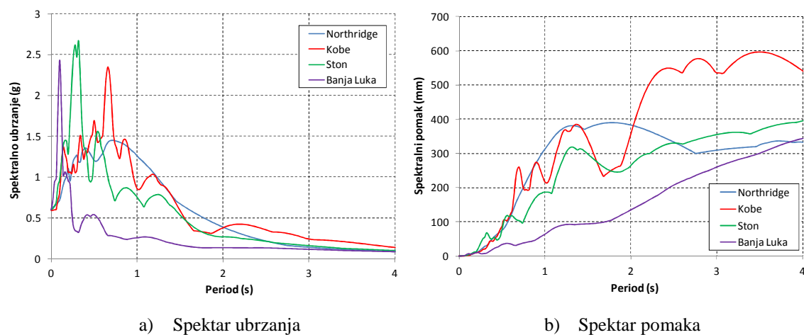
Slika 3.28. Spektar ubrzanja i pomaka za usvojene akcelelograme realnih potresa
