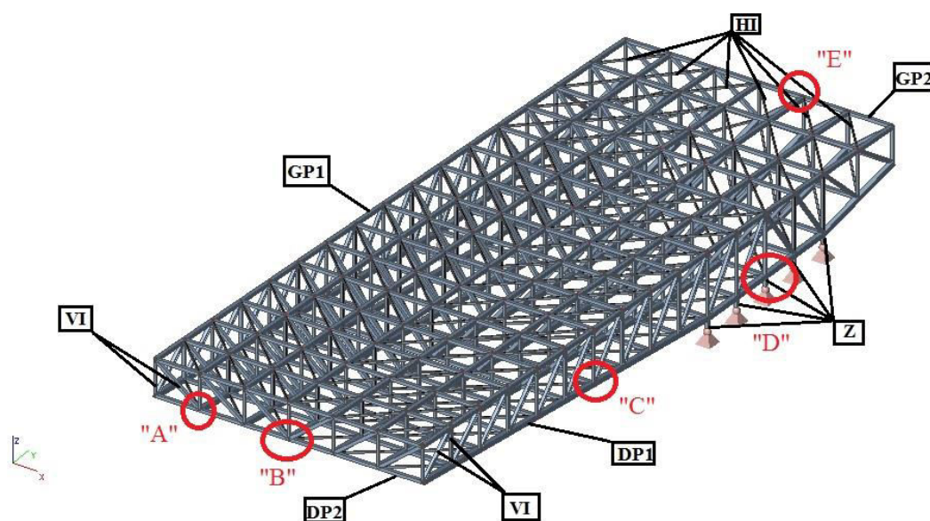
Slika 6.1 Oznake detalja proračunatih priključaka
