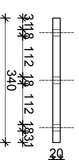
presjek kroz P1
