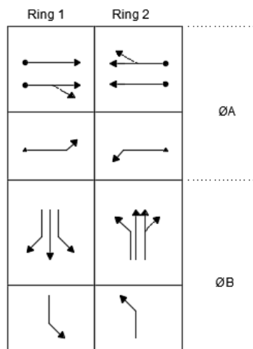
Slika 2.10. Ring dijagram
