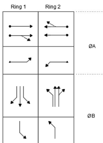
Slika 2.10. Ring dijagram
