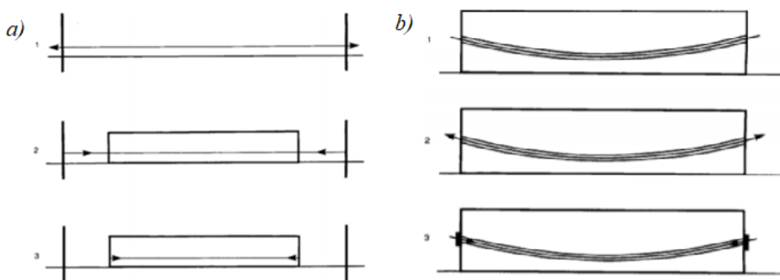
Slika 2.3 Načini prednapinjanja a) Prethodno prednapinjanje b) Naknadno (kabelsko) prednapinjanje [3]
