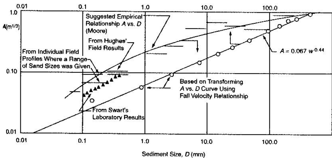
Slika 6.2. Dean-ov dijagram
