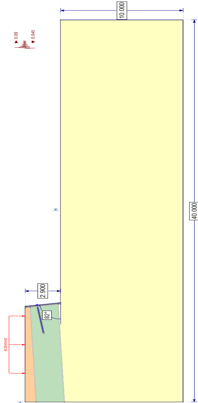
Slika 21. Model za stabilnost pokosa
