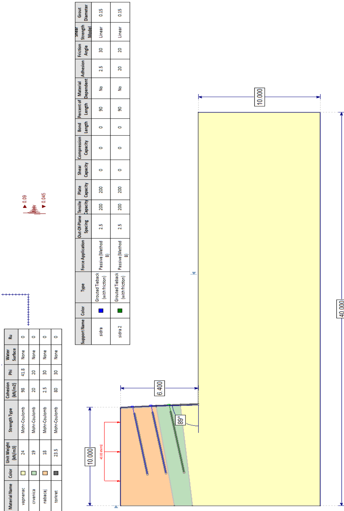
Slika 7. Model za stabilnost pokosa
