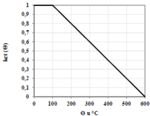
Slika 3.2. Koeficijent k_c(\theta) kojim se uzima u obzir umanjenje vlačne čvrstoće betona, f_{ctk} , pri povišenim temperaturama [5]
