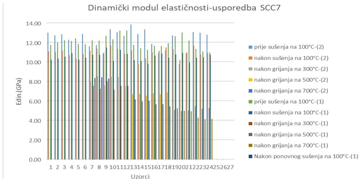
Slika 6.38. Usporedba dinamičkog modula elastičnosti uzoraka hladjenih vodom i na zraku; a) SCC5; b) SCC6; c) SCC7
