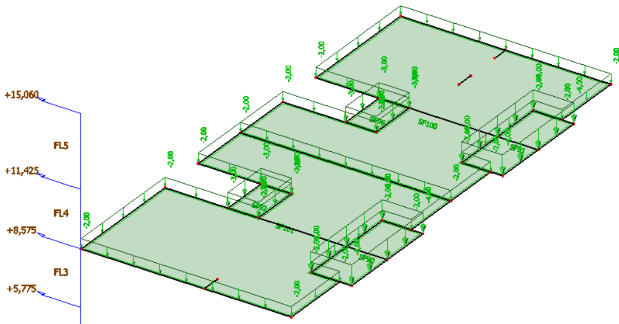
Slika 29: pokretno opterećenje(q)
