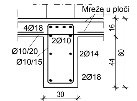
Presjek D-D
