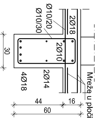
Presjek C-C
