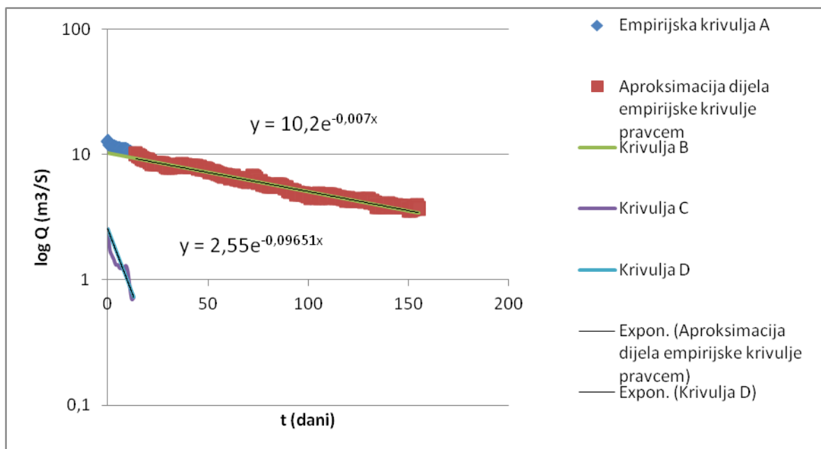
5.55. Aproximacija krivulje recesije za rijeku Rudu u razdoblju od 24.4. – 28.9.2003.(polu-logaritamsko mjerilo)
