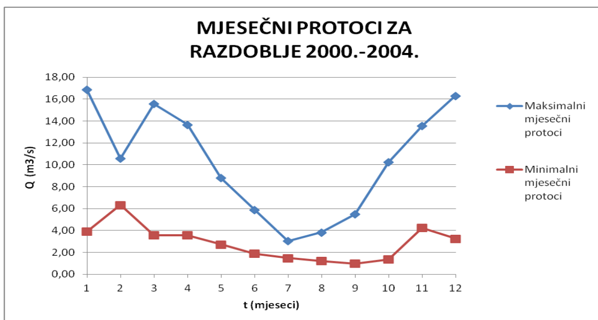
3.8. Prikaz minimalnih i maksimalnih mjesečnih protoka za razdoblje 2000.-2004
