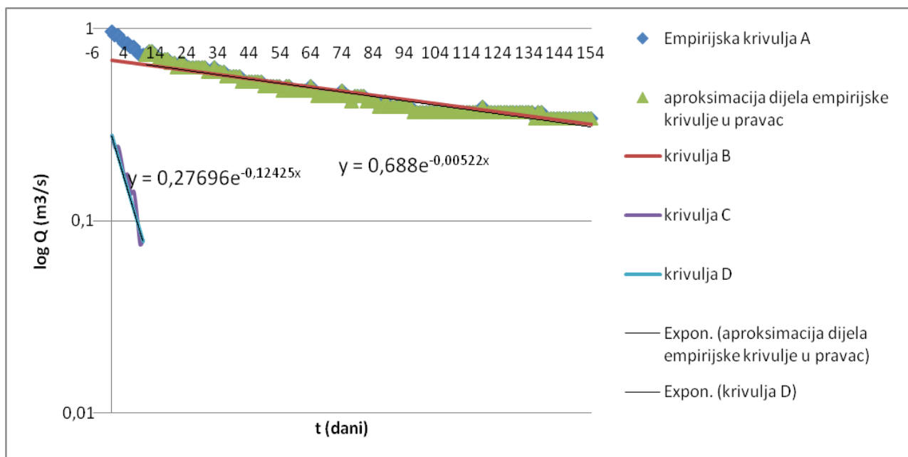
5.69. Aproximacija krivulje recesije za rijeku Žrnovnicu u razdoblju od 26.4. – 30.9.2000.(polu-logaritamsko mjerilo)
