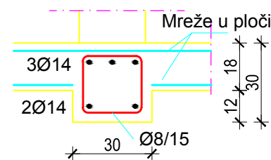
Presjek B-B:
