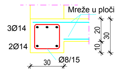
Presjek B-B:
