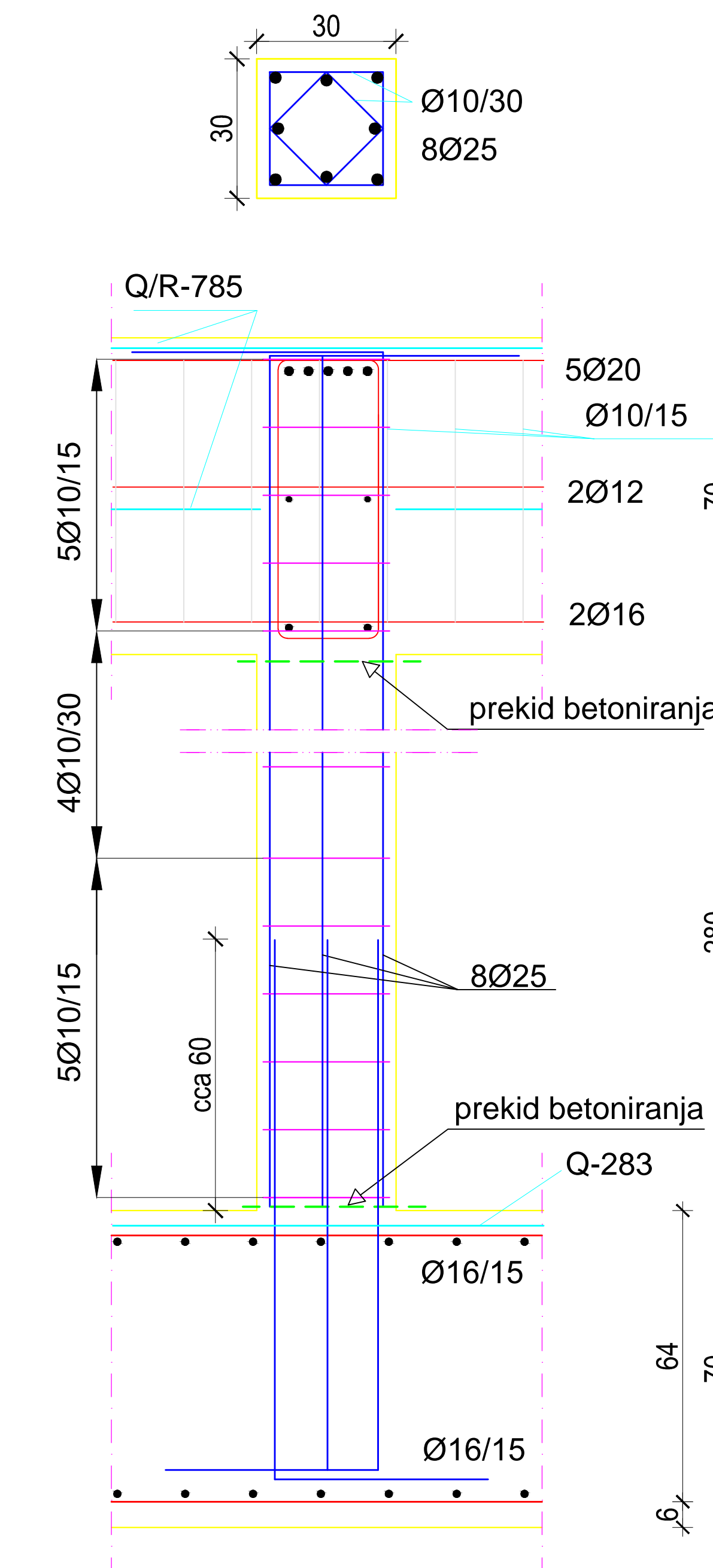
Presjek B-B:
