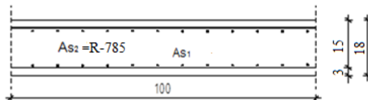
Slika 41. Skica armature ploče na ležaju
