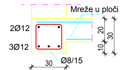
Presjek C-C:
