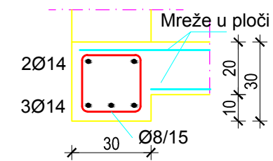
Presjek B-B:
