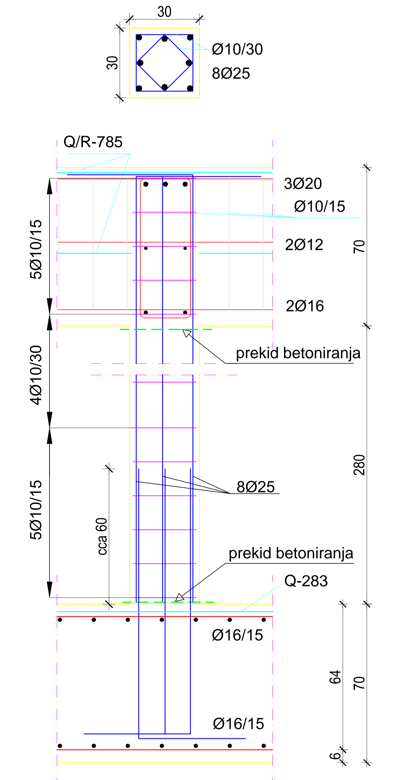
Presjek D-D:
