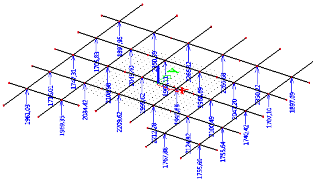
Slika 146. Dijagram maksimalne uzdužne sile N (kN) za stupove uobičajenu kombinaciju opterećenja
