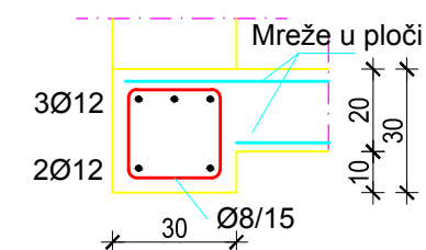
Presjek D-D:
