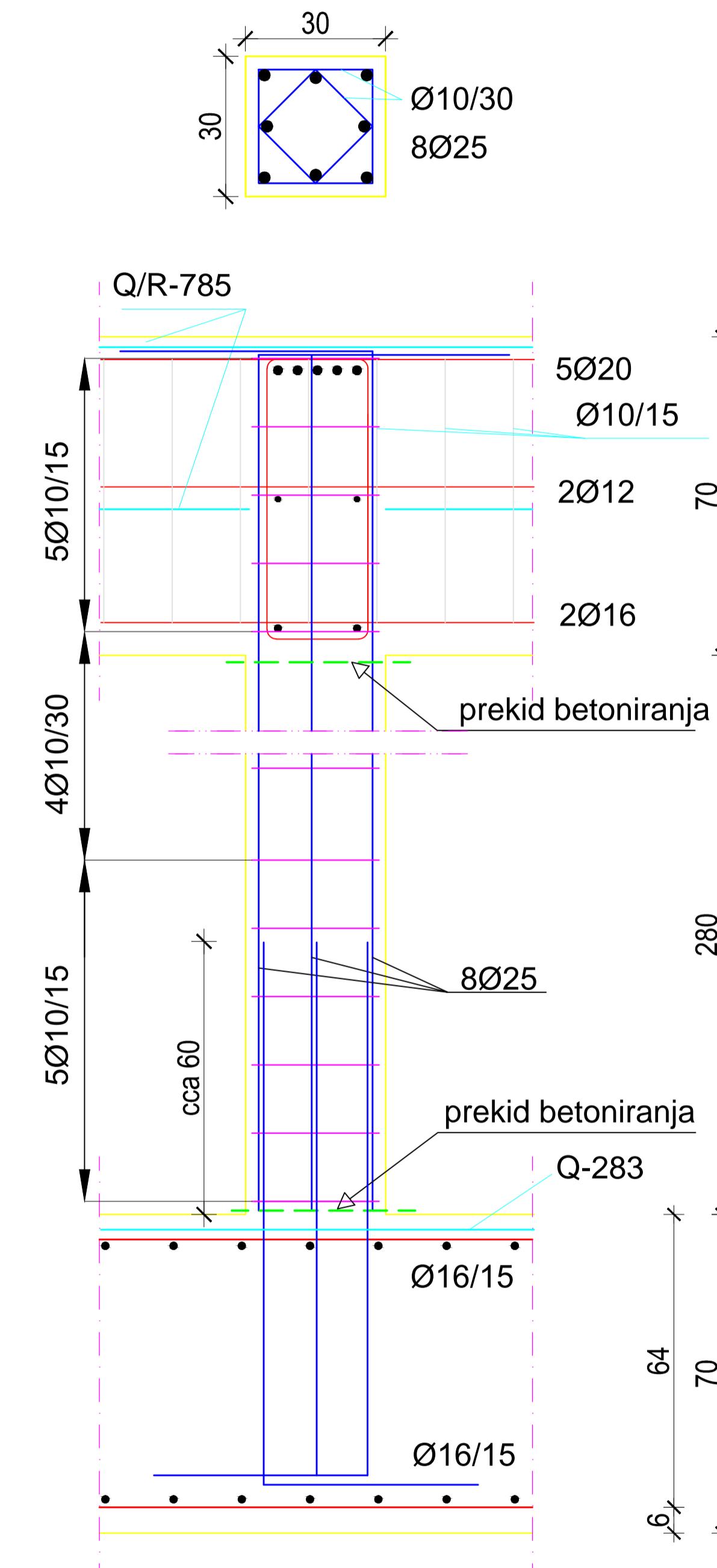
Presjek B-B:
