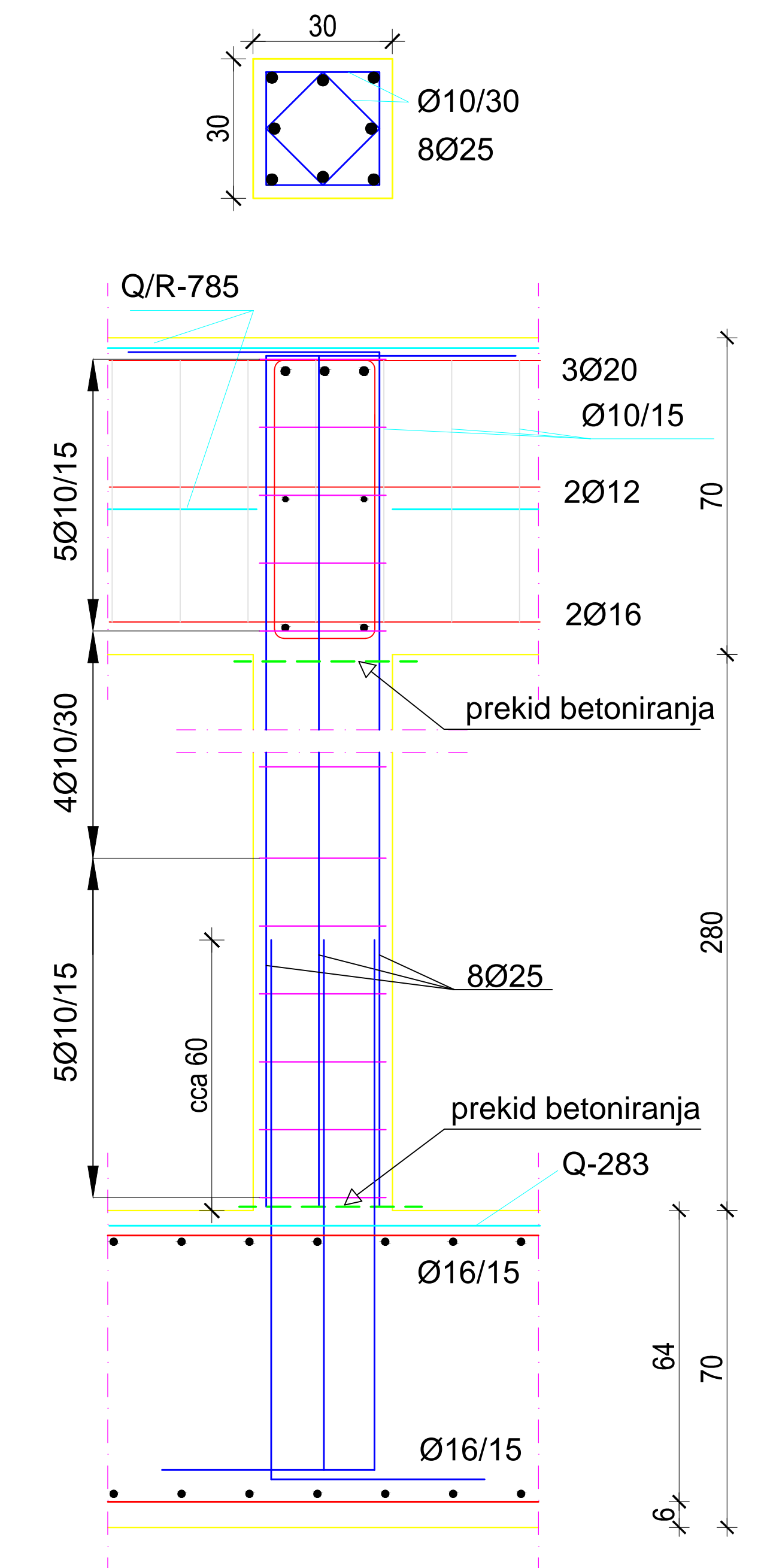
Presjek D-D:
