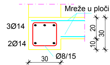
Presjek C-C:
