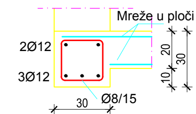
Presjek C-C:
