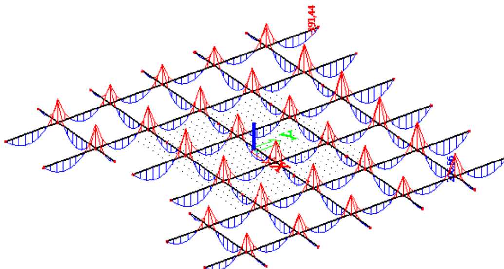
Slika 134. Dijagram momenta savijanja M_y (kNm) za gredu G1B (vlastita težina, dodatno stalno opterećenje "G k ", uporabno opterećenje "Q k ")
