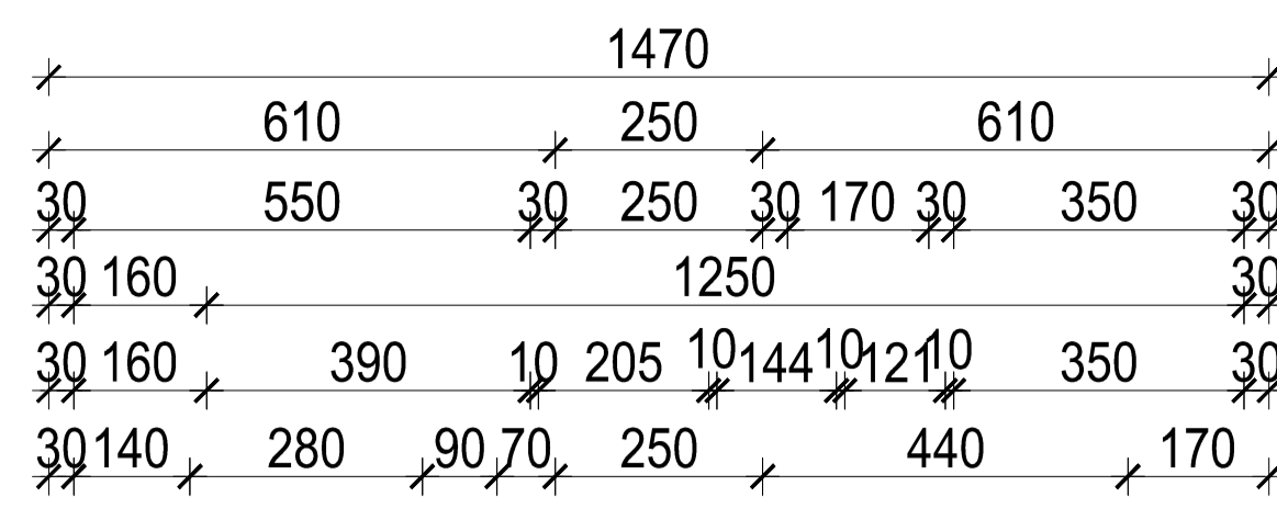
TLOCRT 2. KATA
