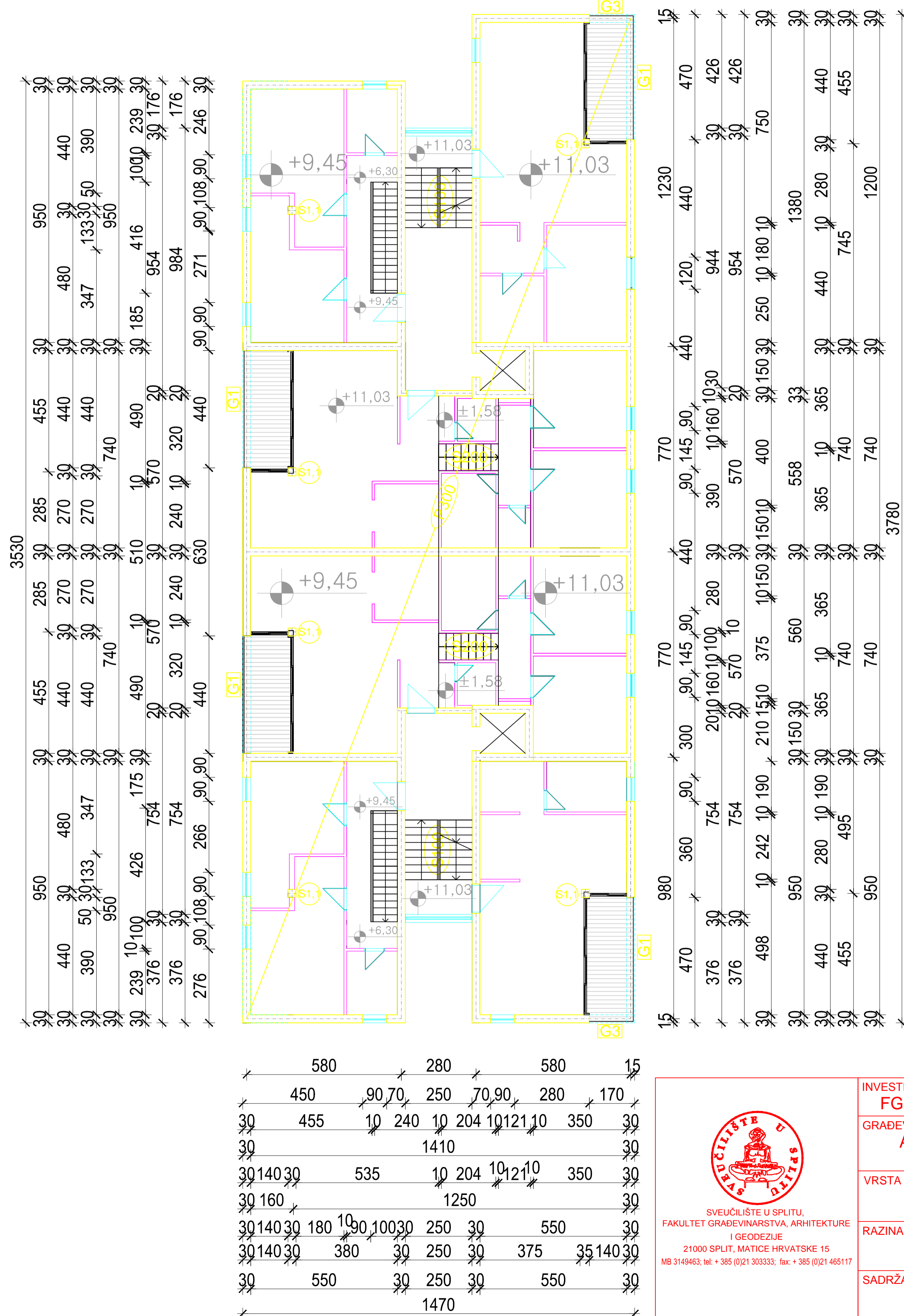
TLOCRT 3. KATA
