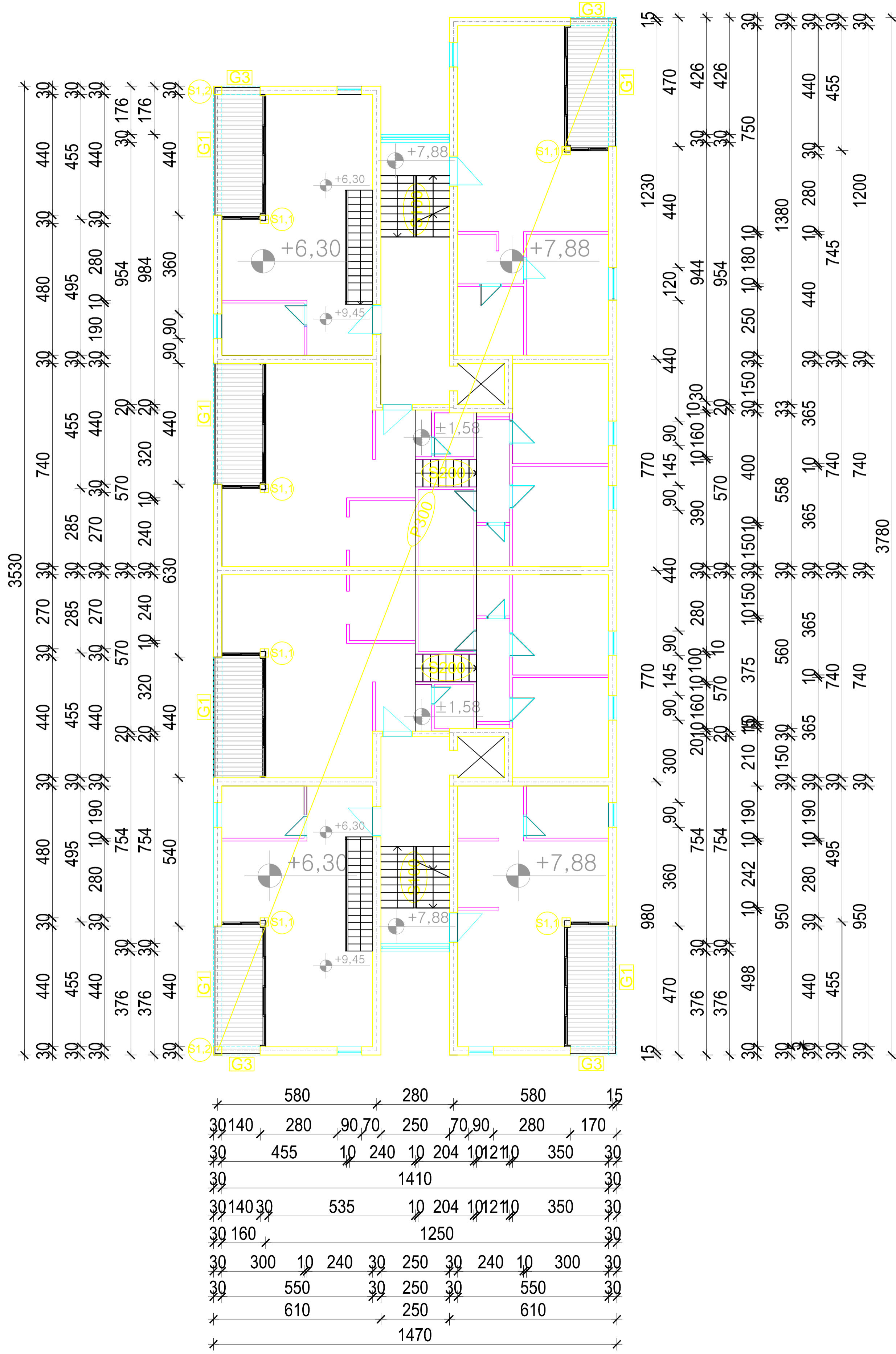
TLOCRT 2. KATA
