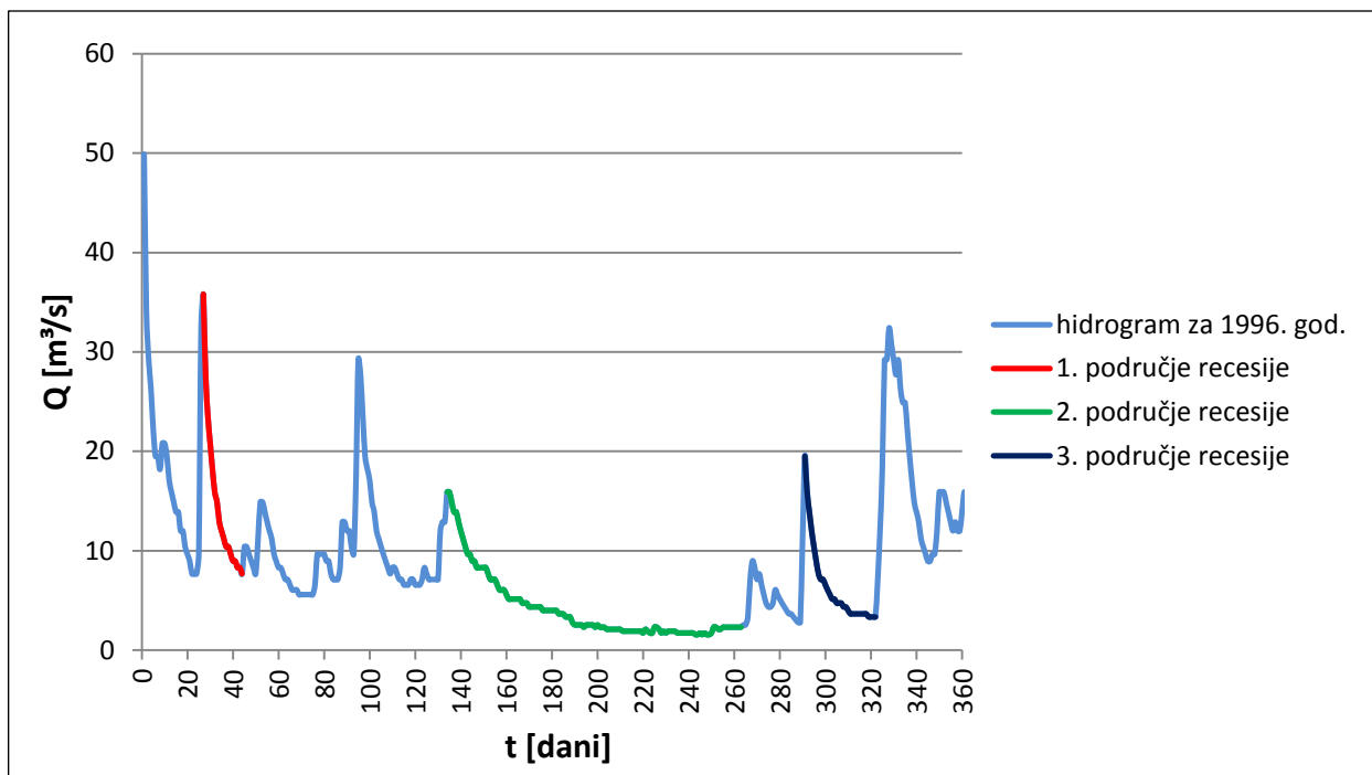
Slika 6.7.: Hidrogram otjecanja rijeke Vrljike za 1996. godinu
