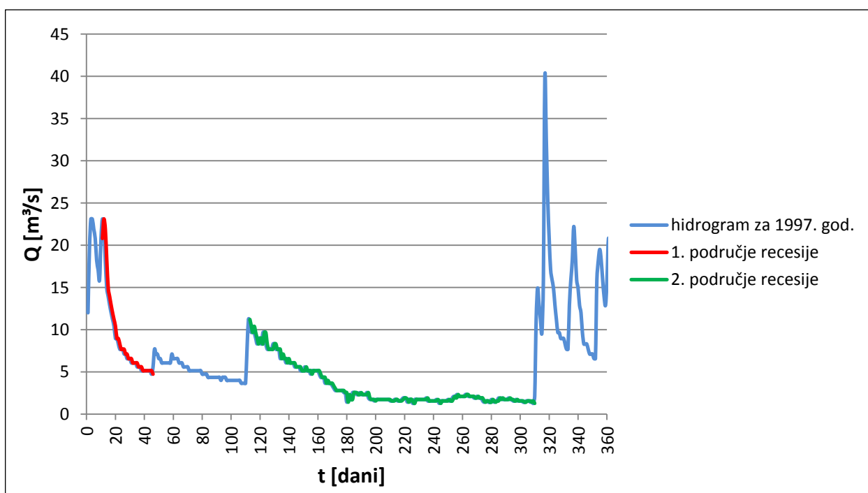
Slika 6.8.: Hidrogram otjecanja rijeke Vrljike za 1997. godinu
