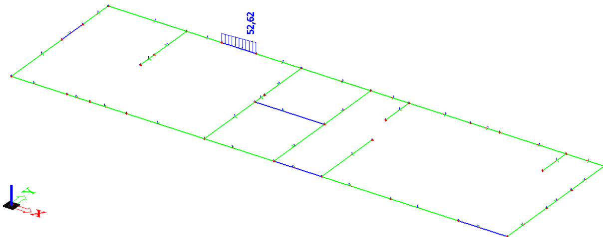
Crtež 8.22. Poprečne sile V_{sd,z} [kN] na gredama za potresnu kombinaciju
