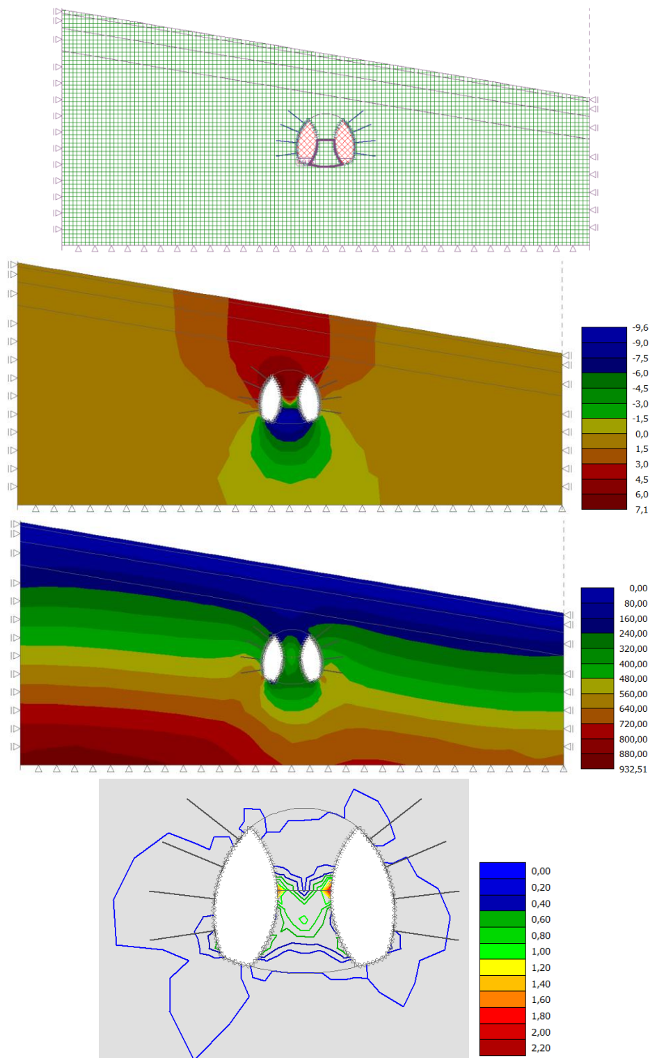
Slika 70.a) Deaktivacija preostalih 30% unutarašnjih sila iz donjeg lijevog dijela; b) Pomaci dz (mm); c) Naprezanja u tlu \sigma_z (kPa); d) Plastične deformacije \epsilon_{pl} (%)
