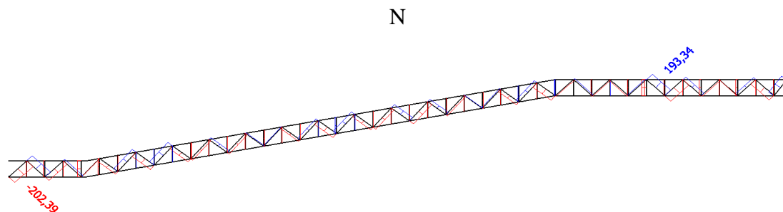
Slika 10.20. Prikaz reznih sila – ispuna glavnog rešetkastog nosača
