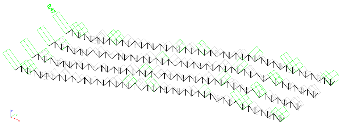
Slika 10.10. Prikaz iskoristivosti ispune glavnog rešetkastog nosača
