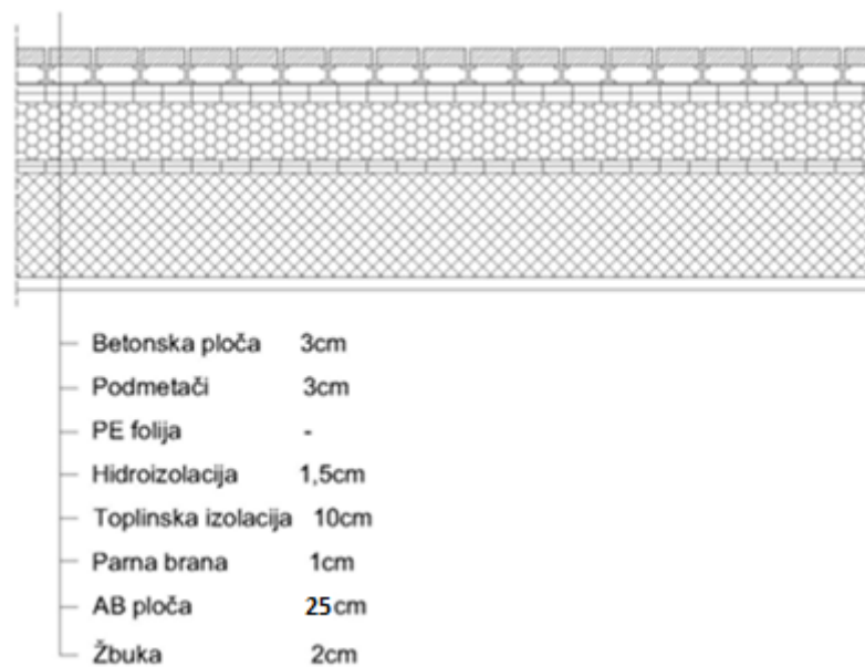
Tablica 8.1 Slojevi ravnog krova
