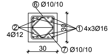
Presjek 2-2
