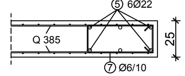
Detalj F
