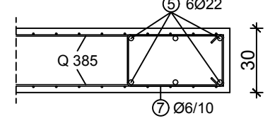
Detalj C
