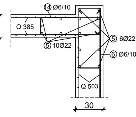
Detalj D
