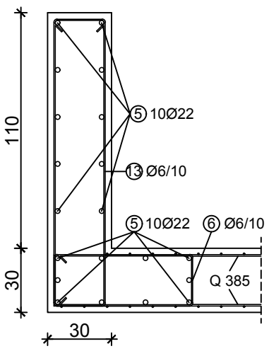
Detalj A
