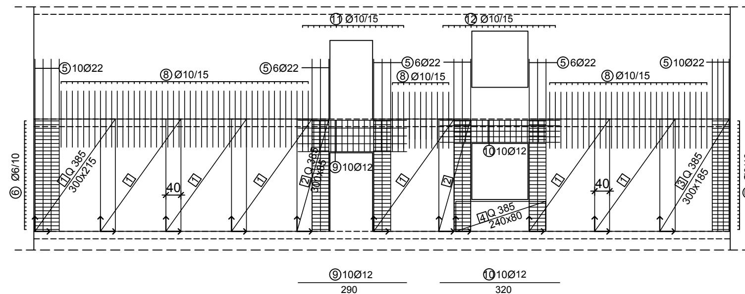
Presjek 1-1
