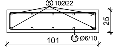
Detalj F
