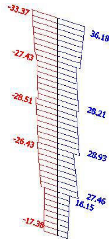
Slika 11.1. Maksimalni moment savijanja M_y za proračun stupa, GSN-K11
