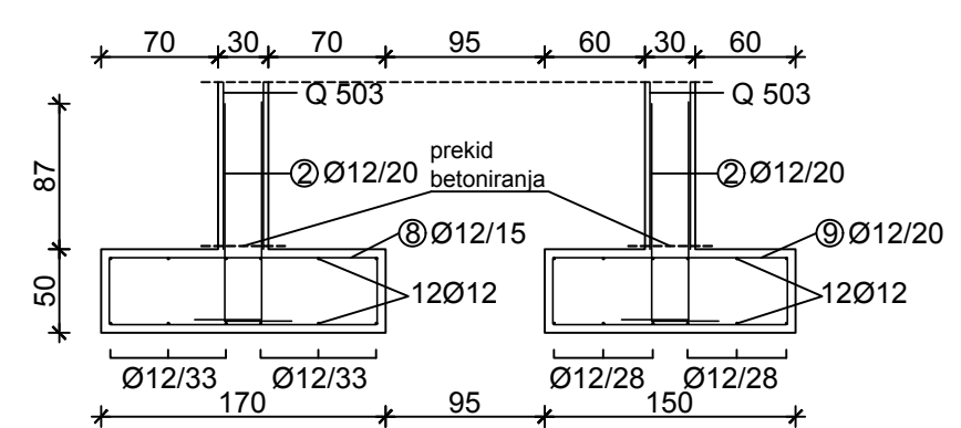
Presjek 7-7
