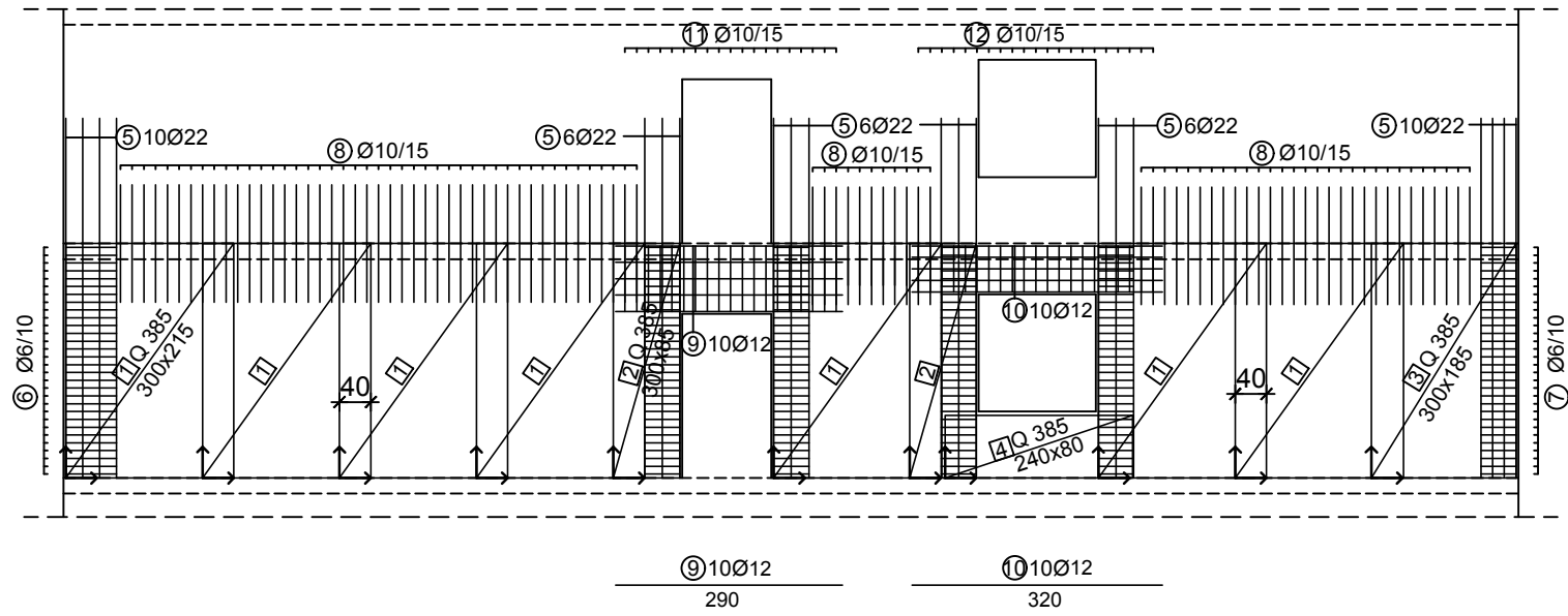
Presjek 1-1
