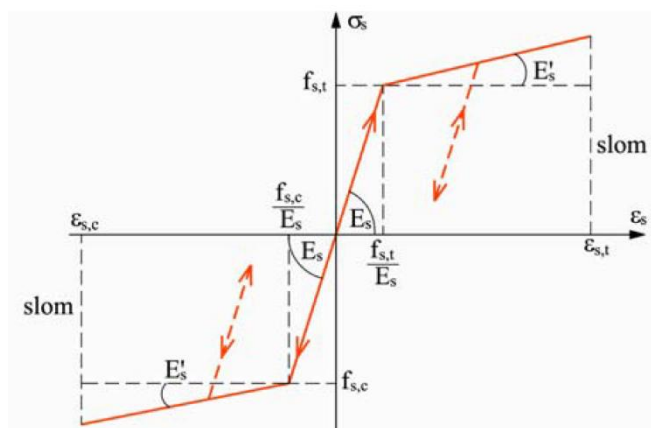
Crtež 3.3. Radni dijagram čelika za armiranje
