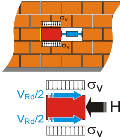
Crtež 2.5. Ispitivanje posmične čvrstoće zida – in situ
