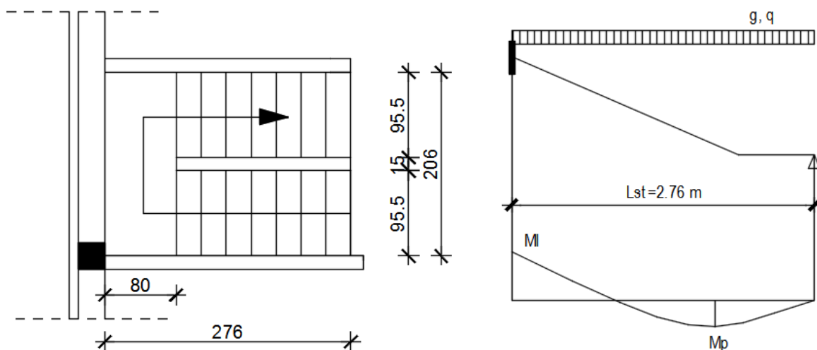
Slika 11.1.1 Tlocrt stubišta
