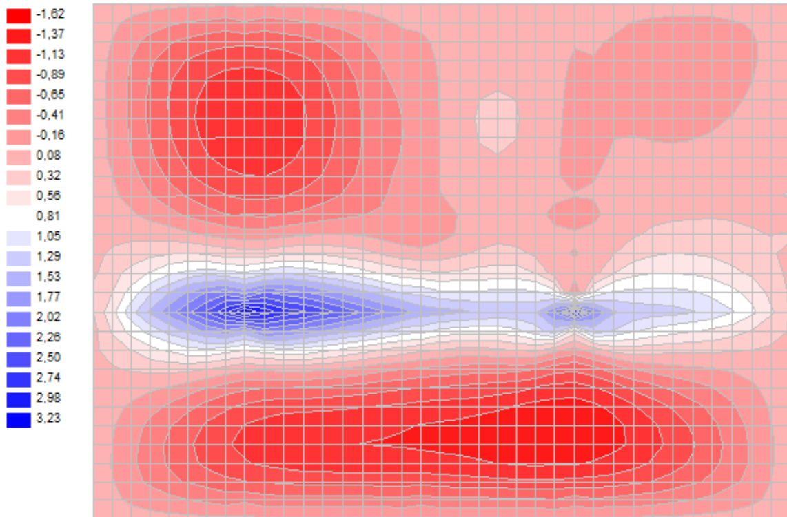
Slika 4.10. Količina potrebne armature M_y ( \text{cm}^2/\text{m}' )
