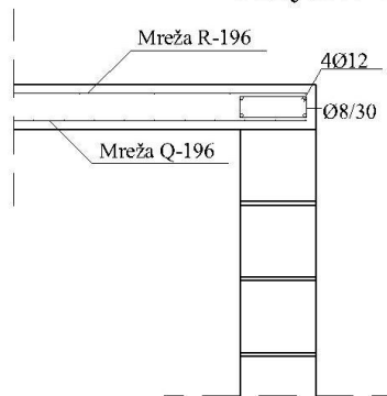
Presjek 1-1
