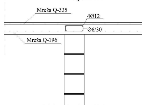
Presjek 2-2
