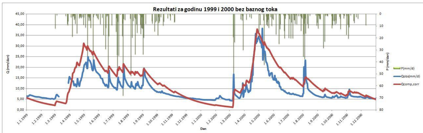
Graf 17: Detaljni rezultati otjecanja za godinu 1999. i 2000. bez baznog toka
