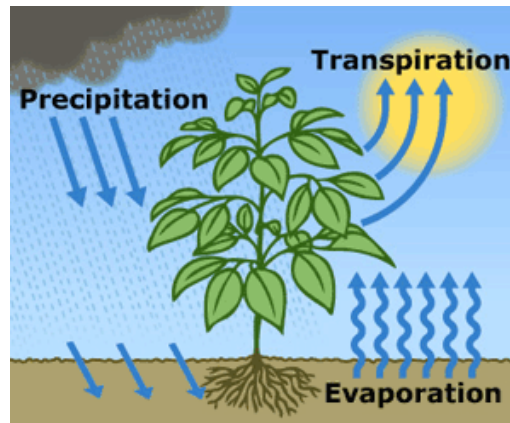
Slika 8: Proces evapotranspiracije
