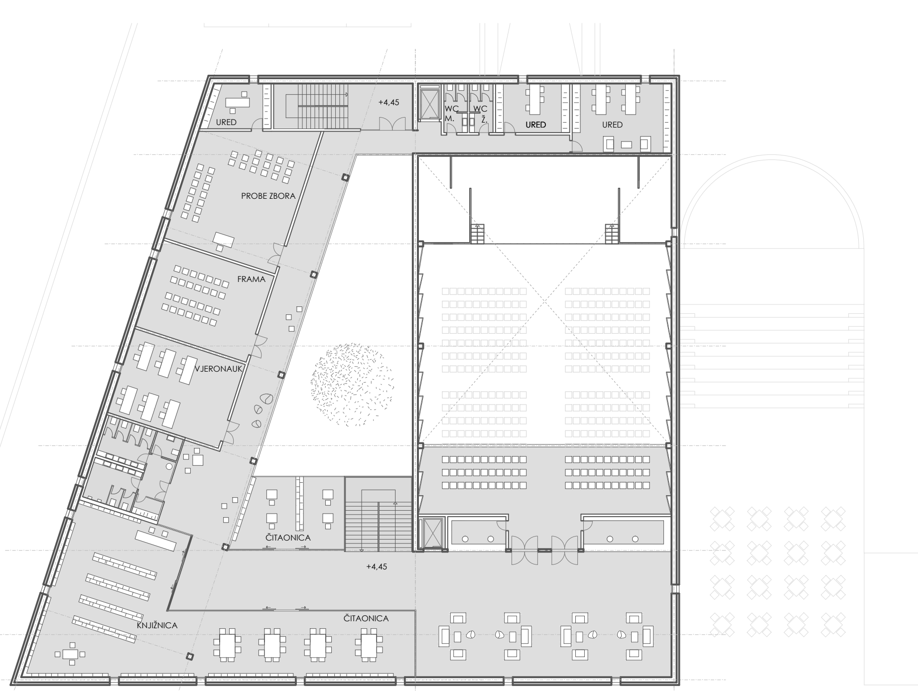
TLOCRT KAT
