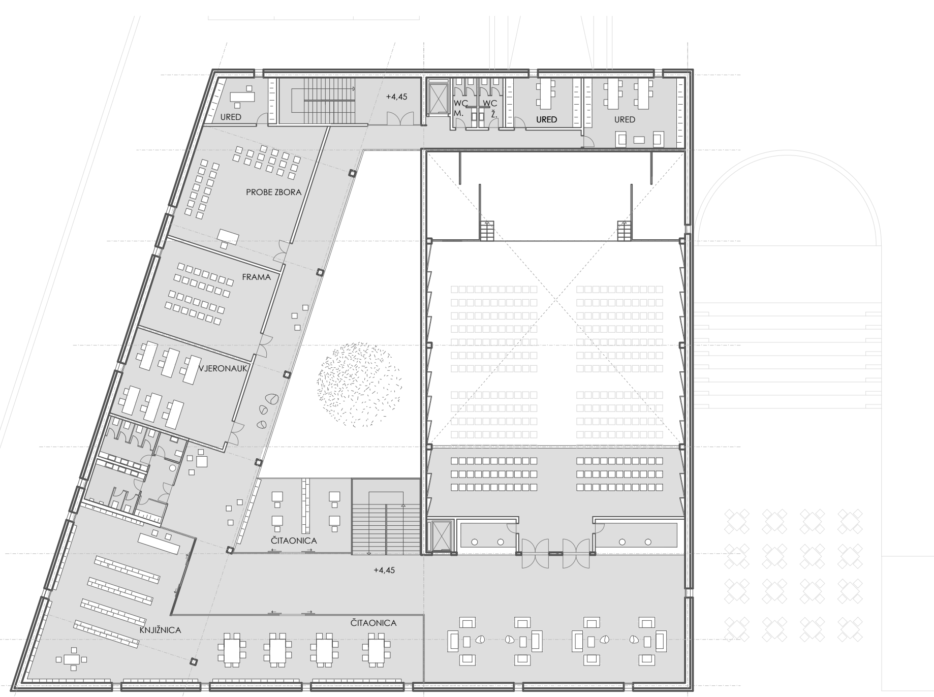
TLOCRT KAT
