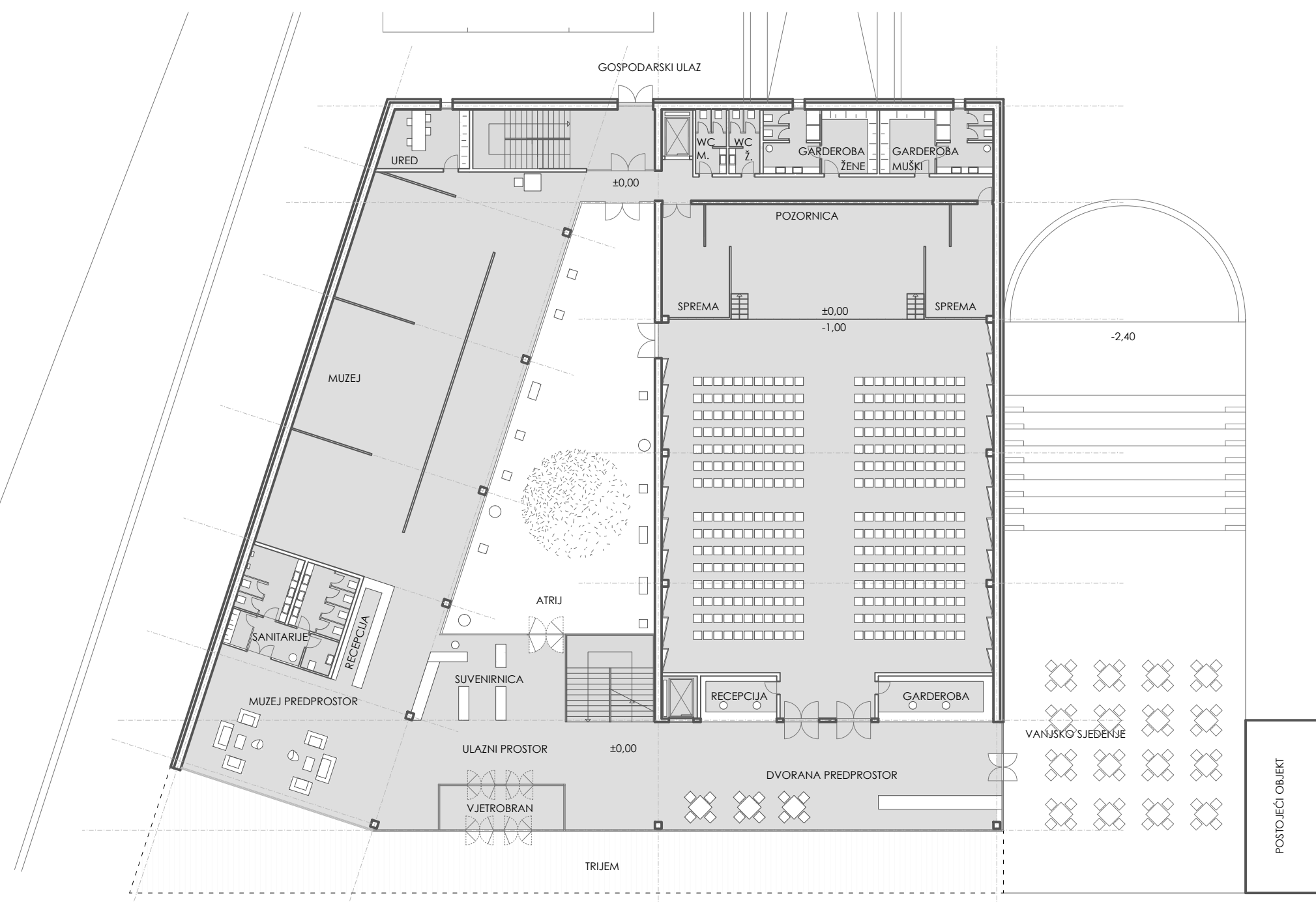
TLOCRT PRIZEMLJE
