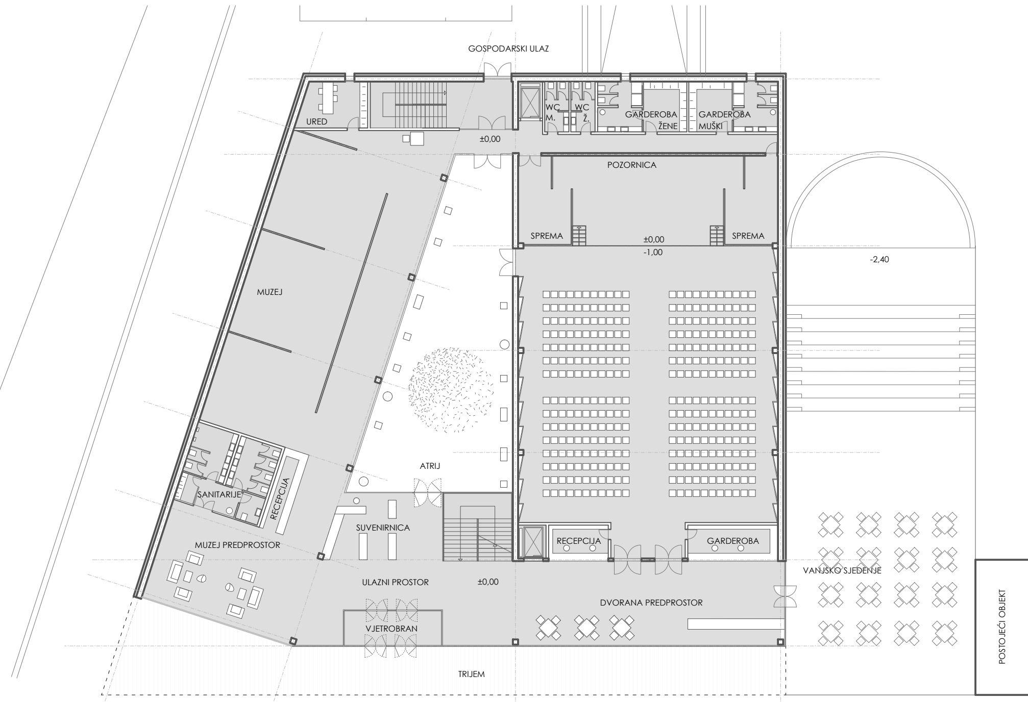
TLOCRT PRIZEMLJE
