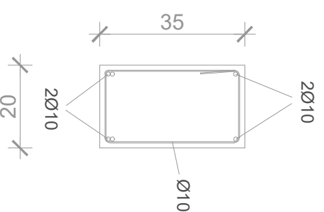
1:25 POPREČNI PRESJEK 2-2
