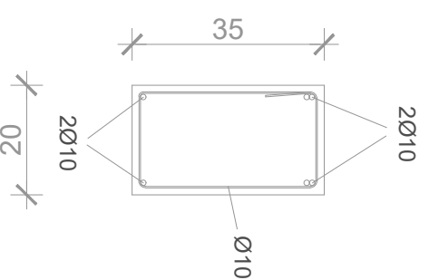
1:25 POPREČNI PRESJEK 3-3
