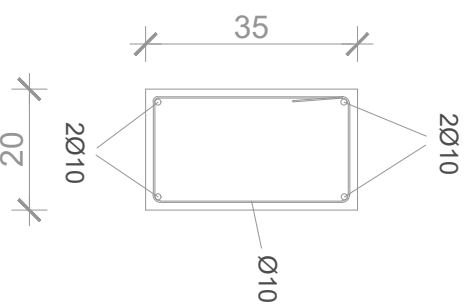
1:25 POPREČNI PRESJEK 1-1
