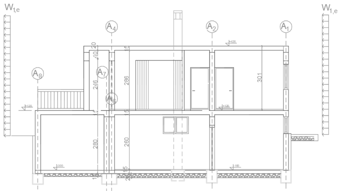
Slika 3.9. Opterećenje vjetrom
