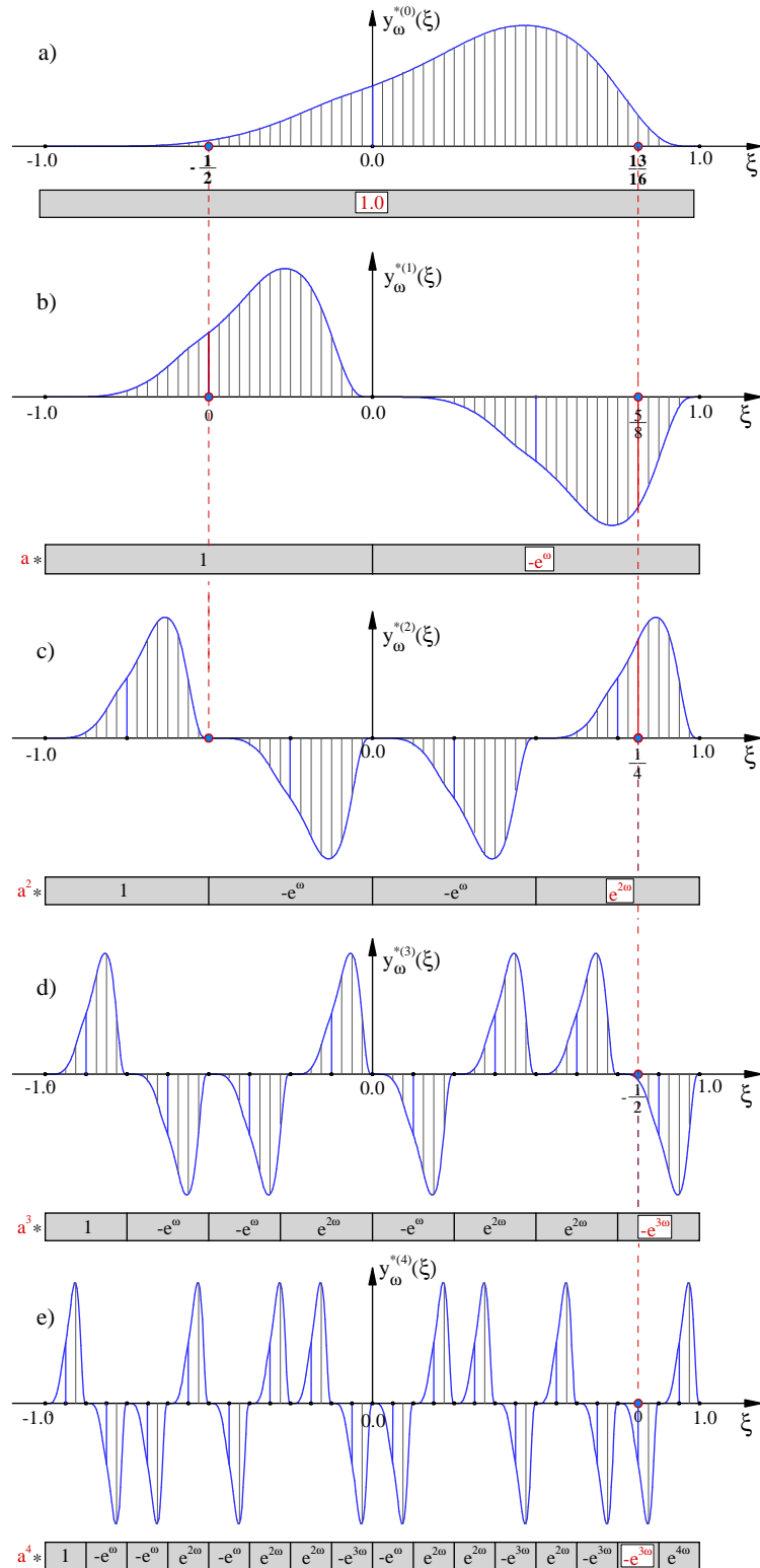
Crtež 5.3 Komponente za izračun do uključivo četvrtu derivaciju funkcije Eup(\xi, \omega)
