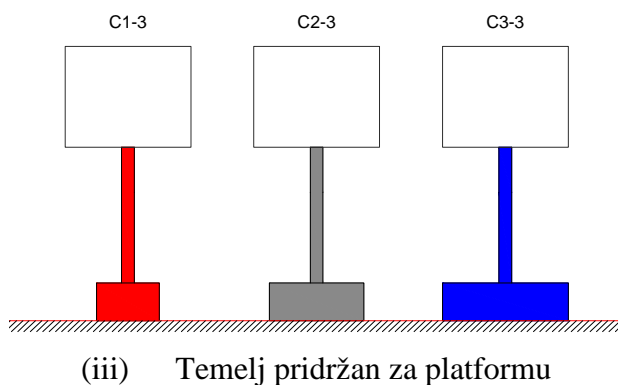
Slika 2.3 Razmatrani načini oslanjanja temelja stupa na dinamičku platformu
