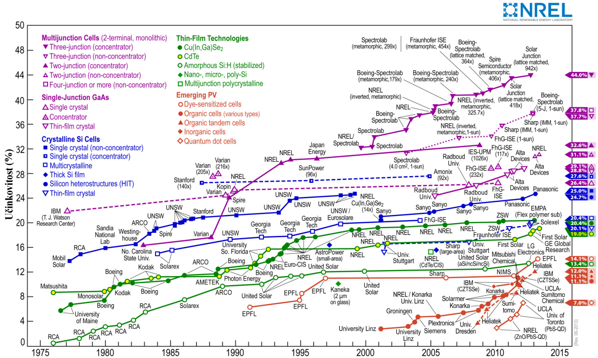
Slika 4.5. Trend povećanja učinkovitosti PV ćelija [T2]
